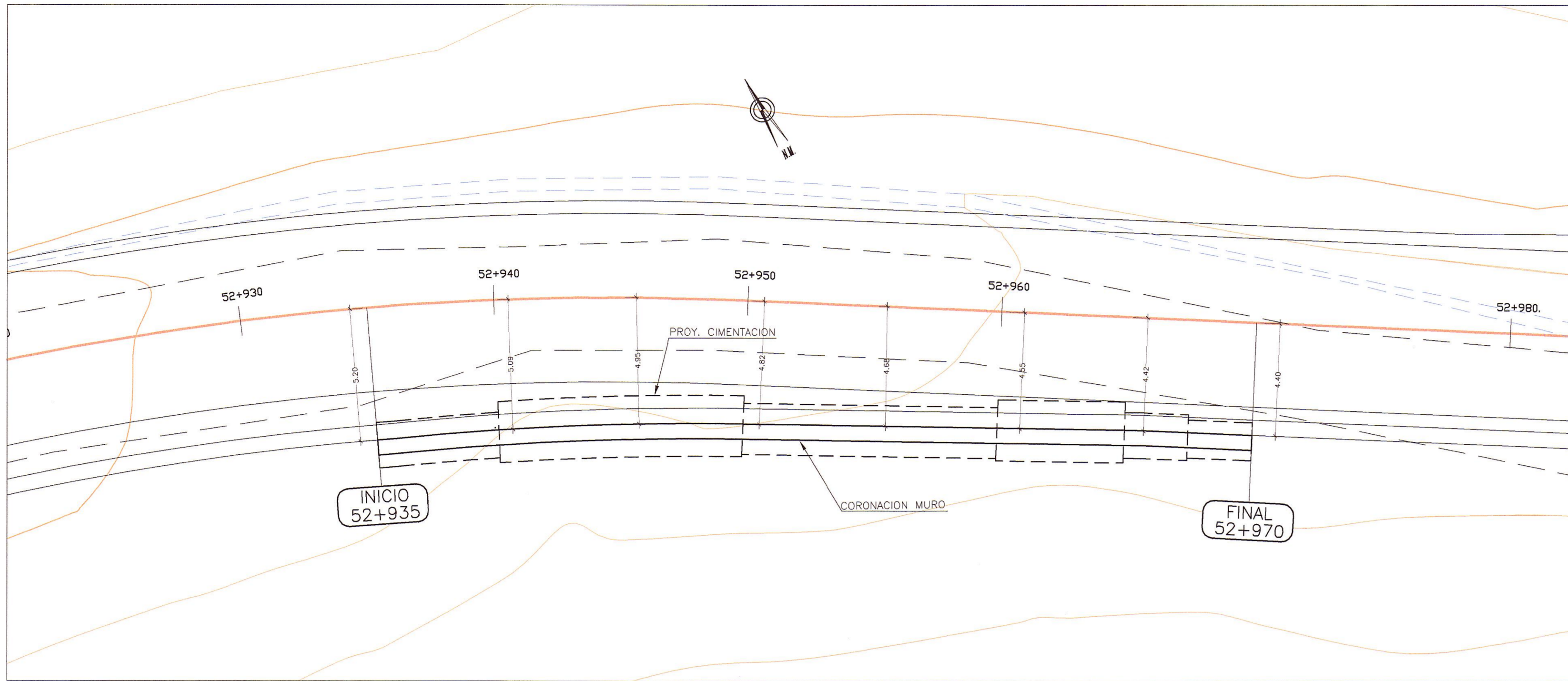
PLANTA ESC. : 1/125
