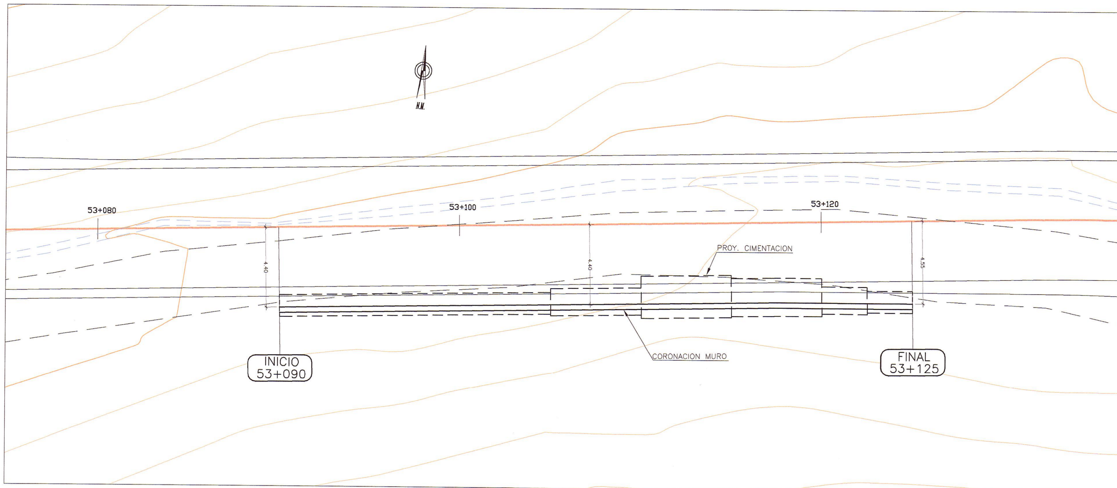
PLANTA ESC.: 1/125
