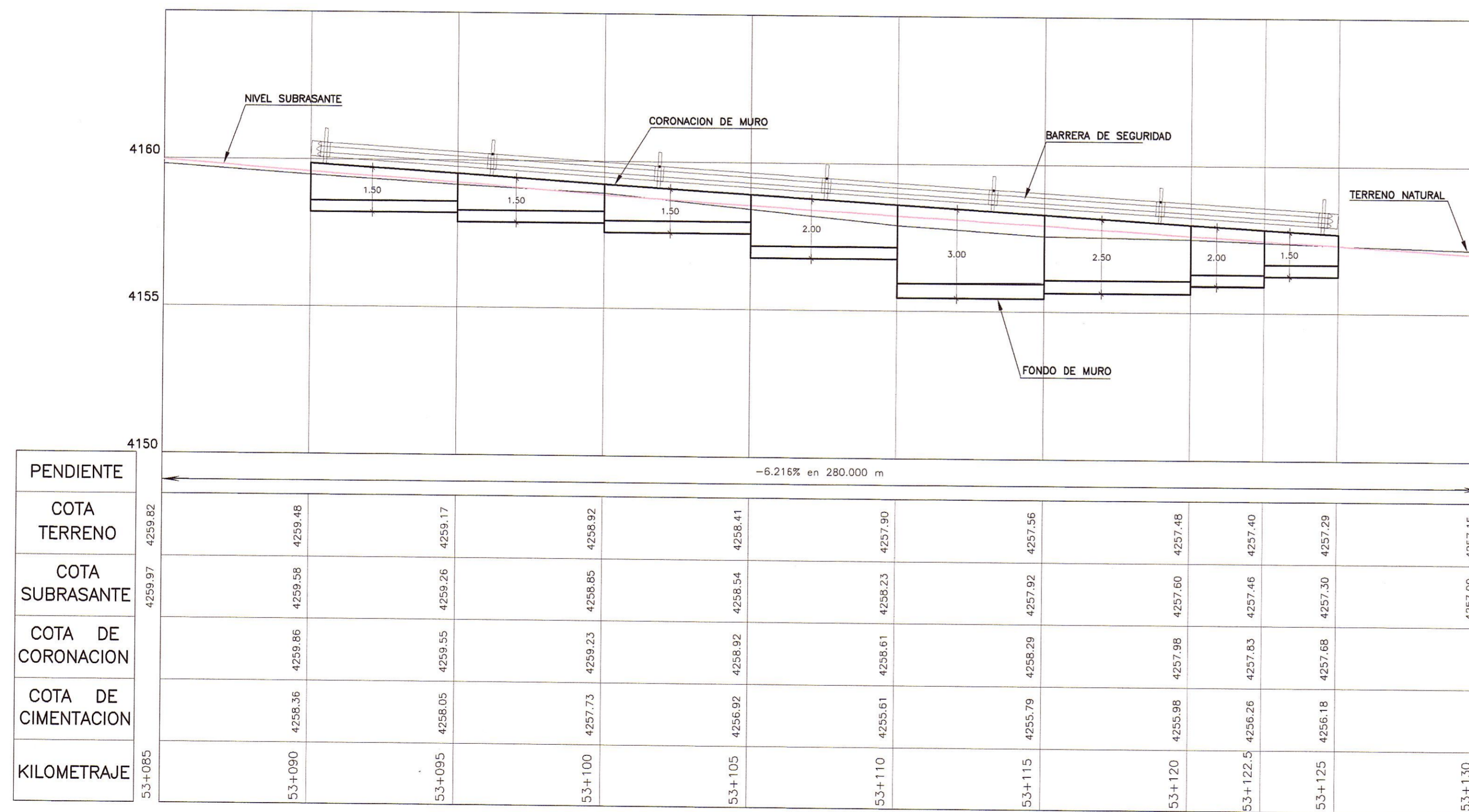
PERFIL LONGITUDINAL
