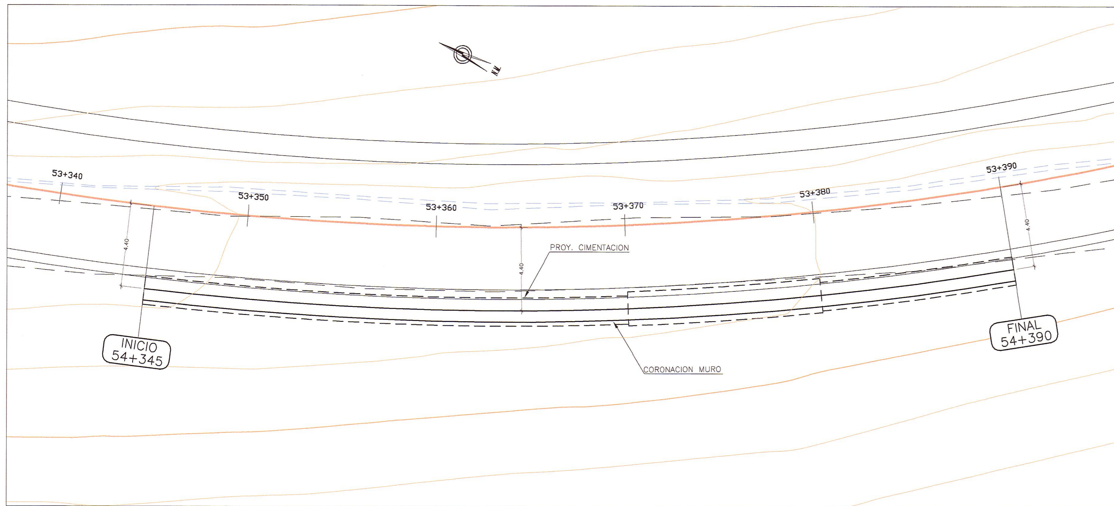
PLANTA ESC. : 1/125
