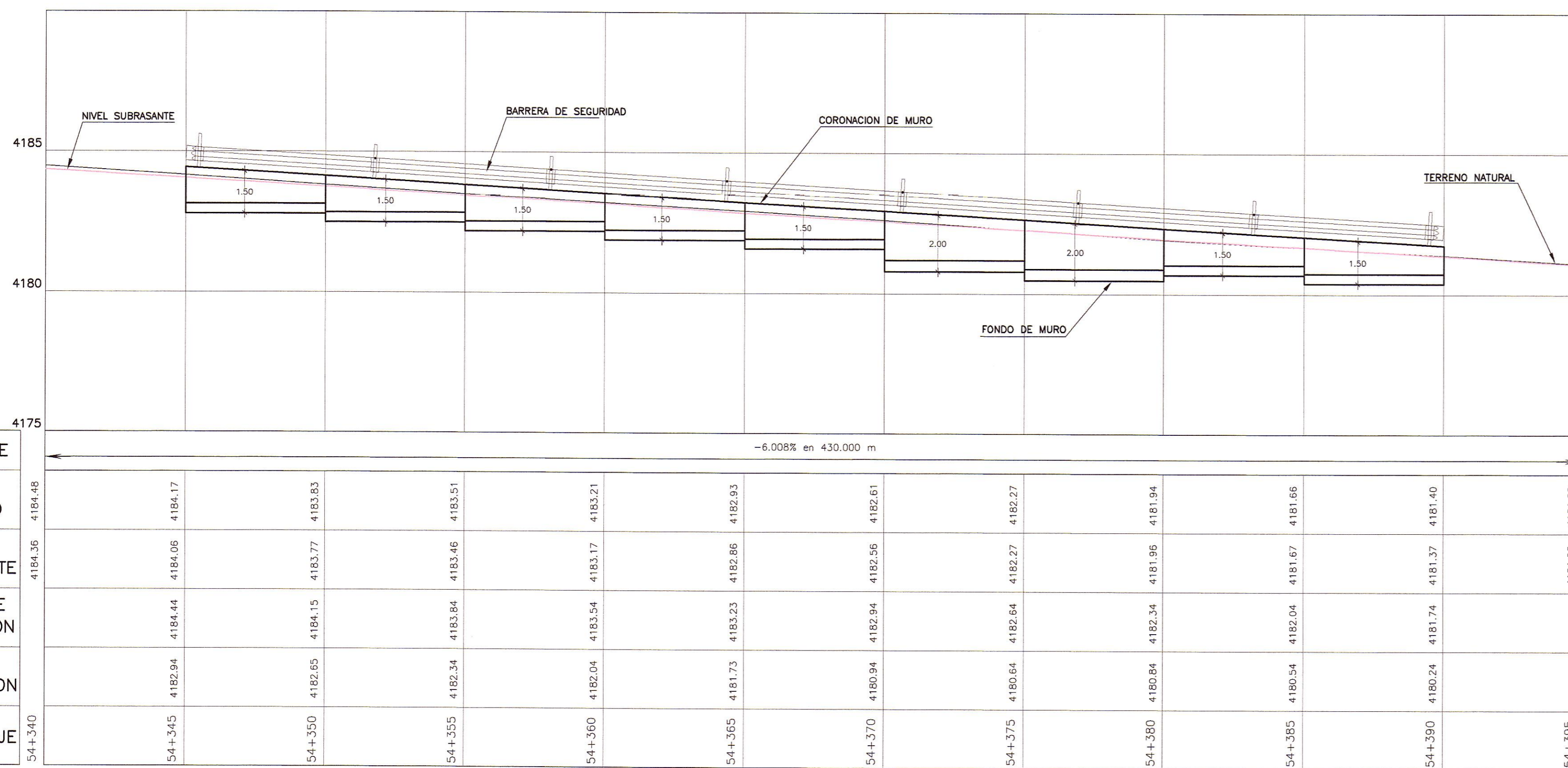
PERFIL LONGITUDINAL
