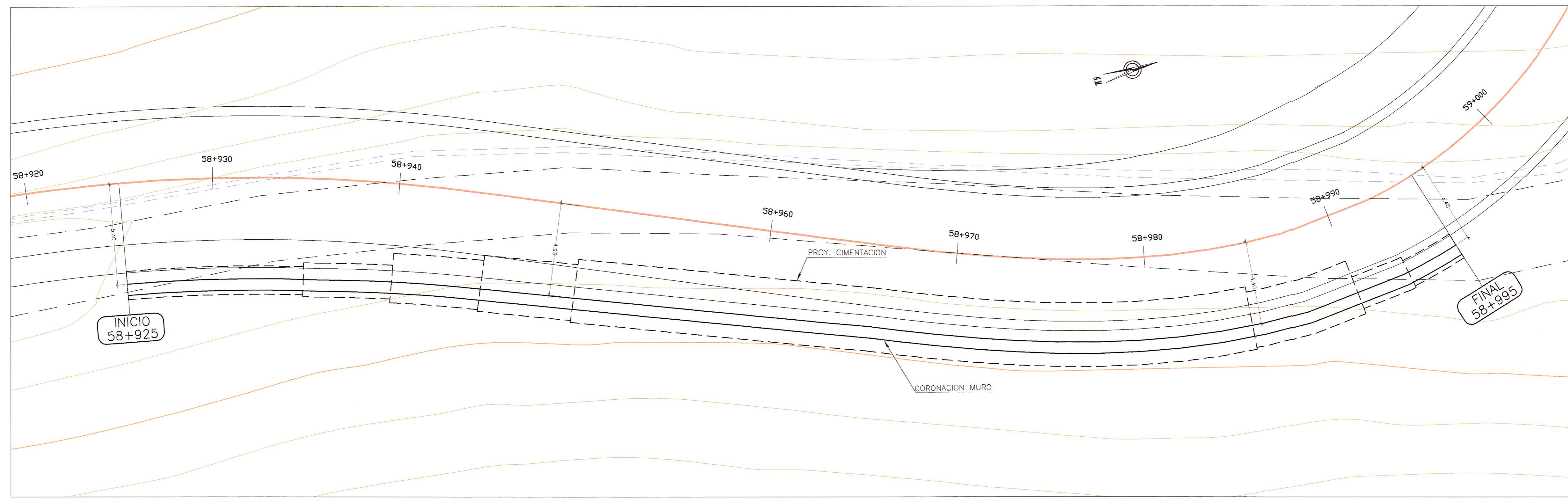
PLANTA ESC.: 1/125
