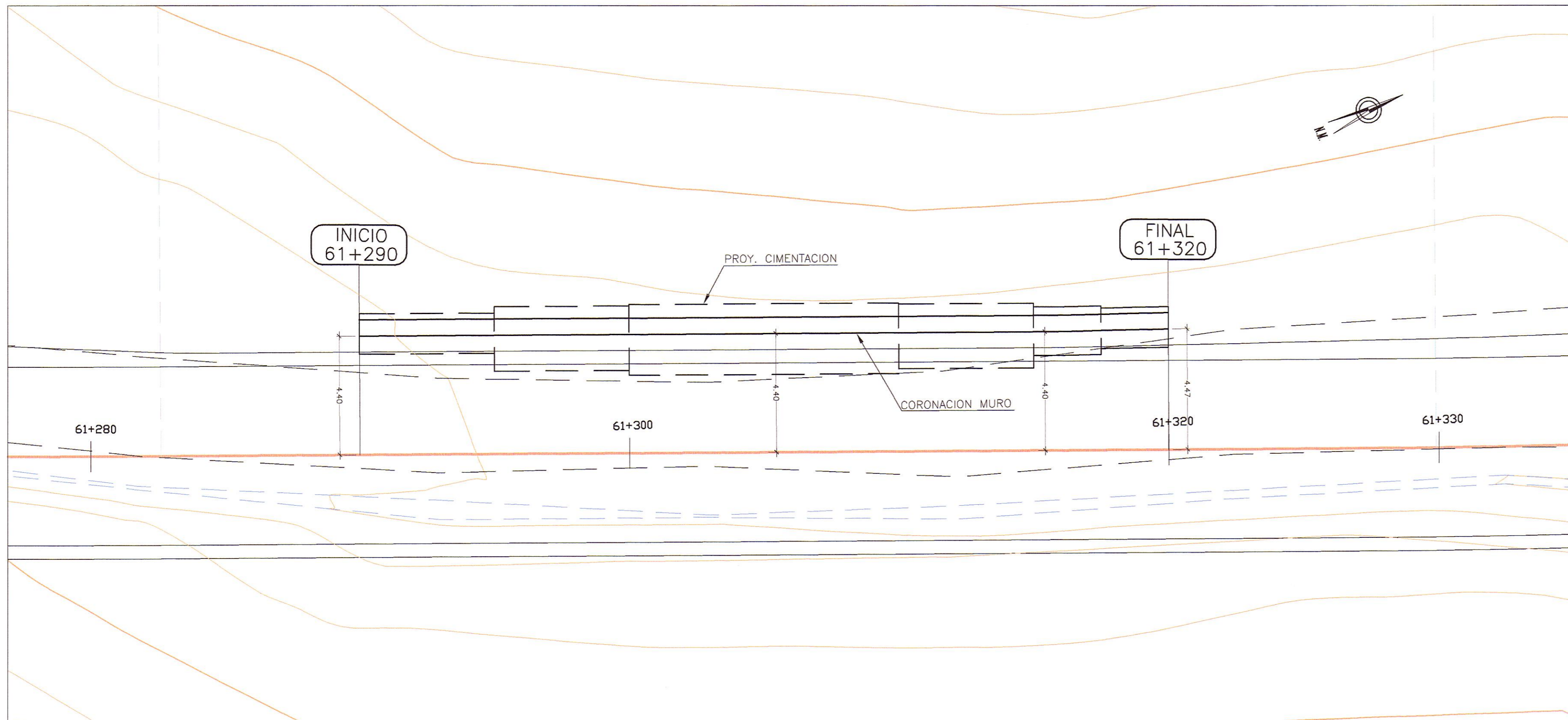
PLANTA Esc. : 1/125
