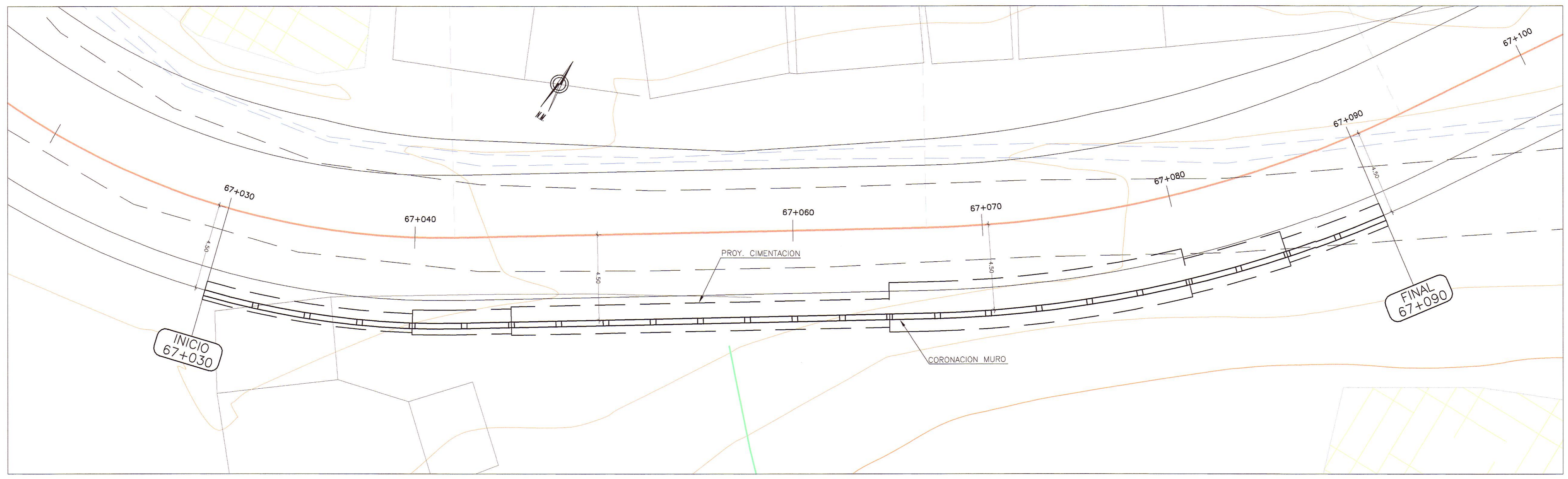
PLANTA ESC. : 1/125
