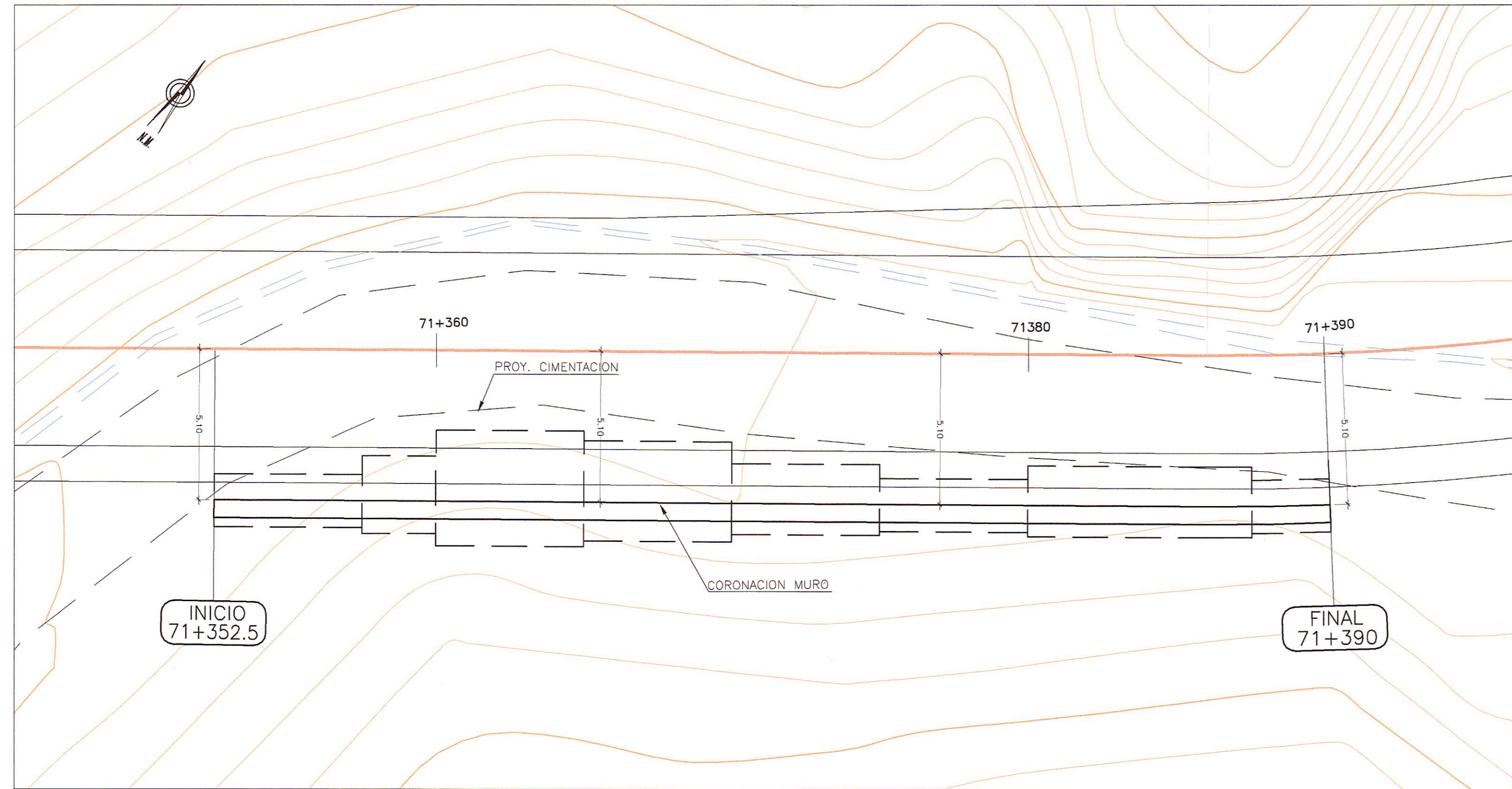
PLANTA ESC. : 1/125
