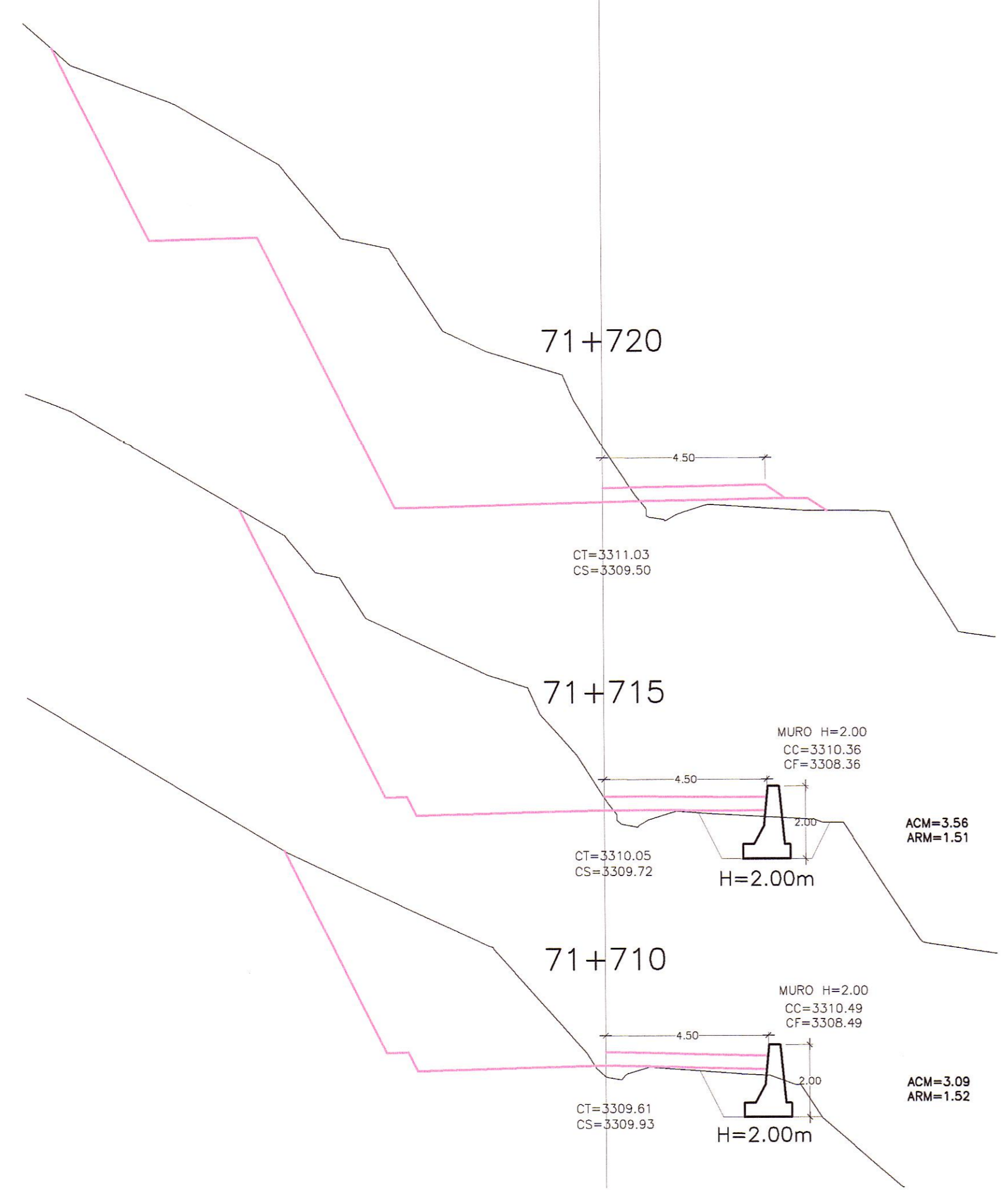
SECCIONES TRANSVERSALES
