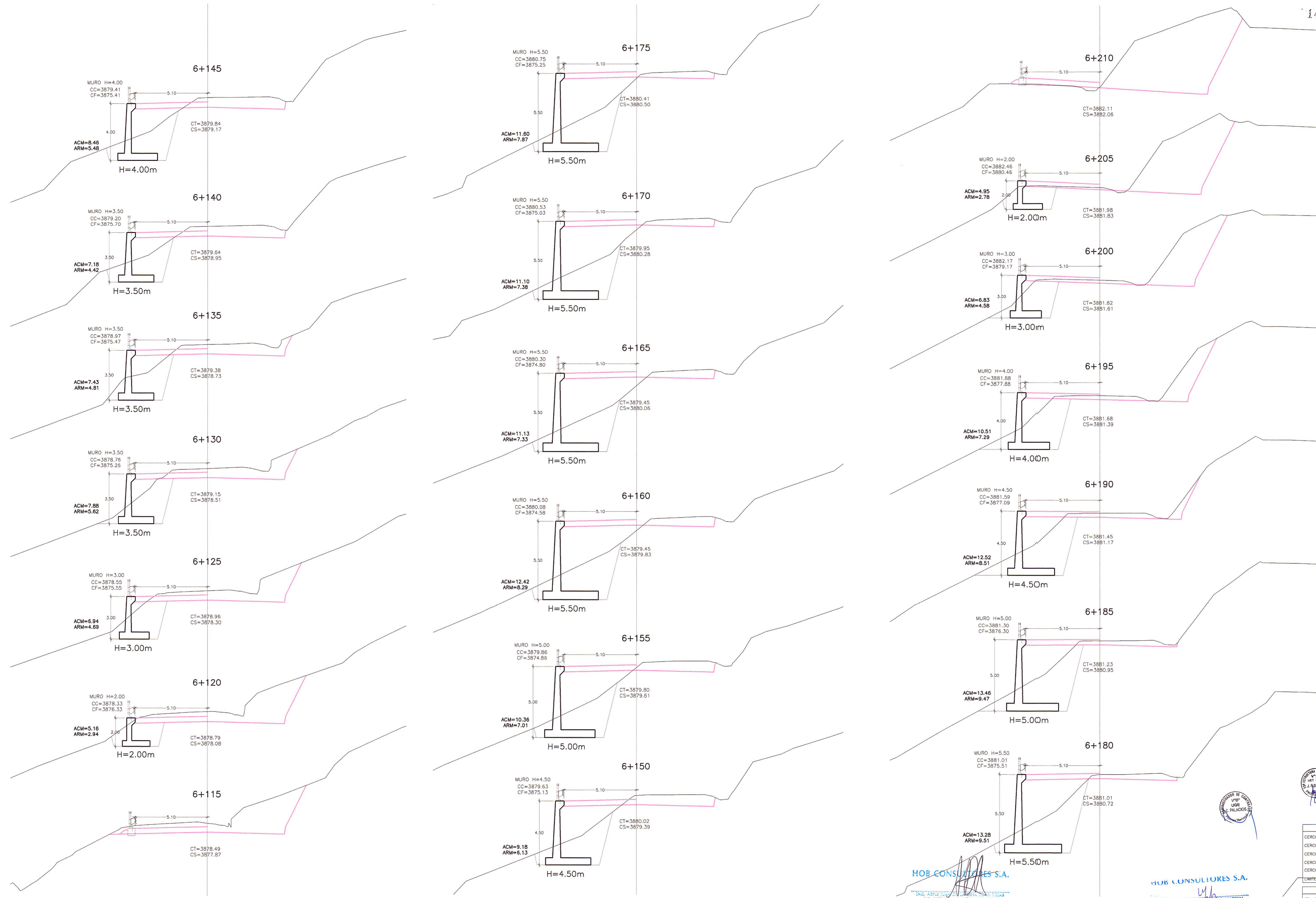
SECCIONES TRANSVERSALES ESC.: 1/125
