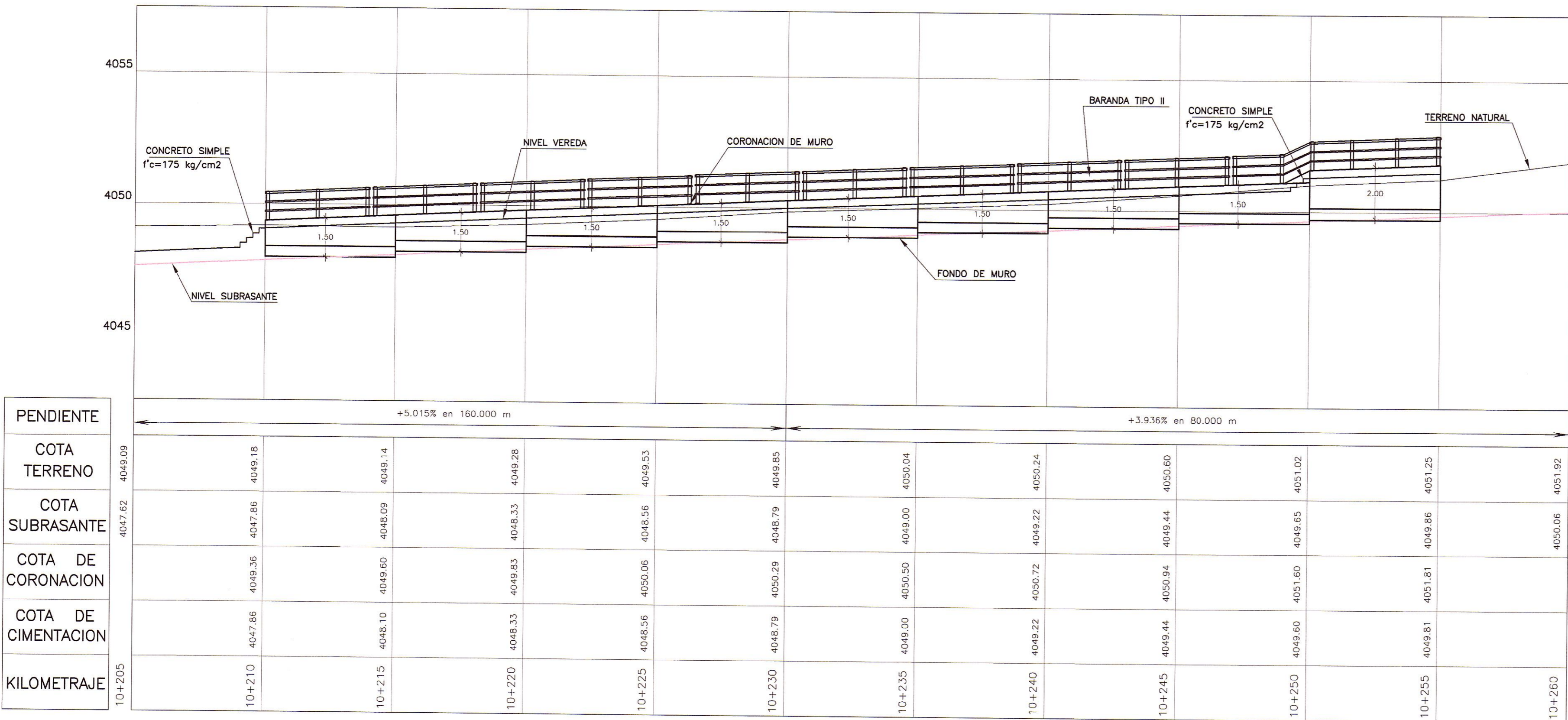
PERFIL LONGITUDINAL ESC. H=1/125 V=1/125
