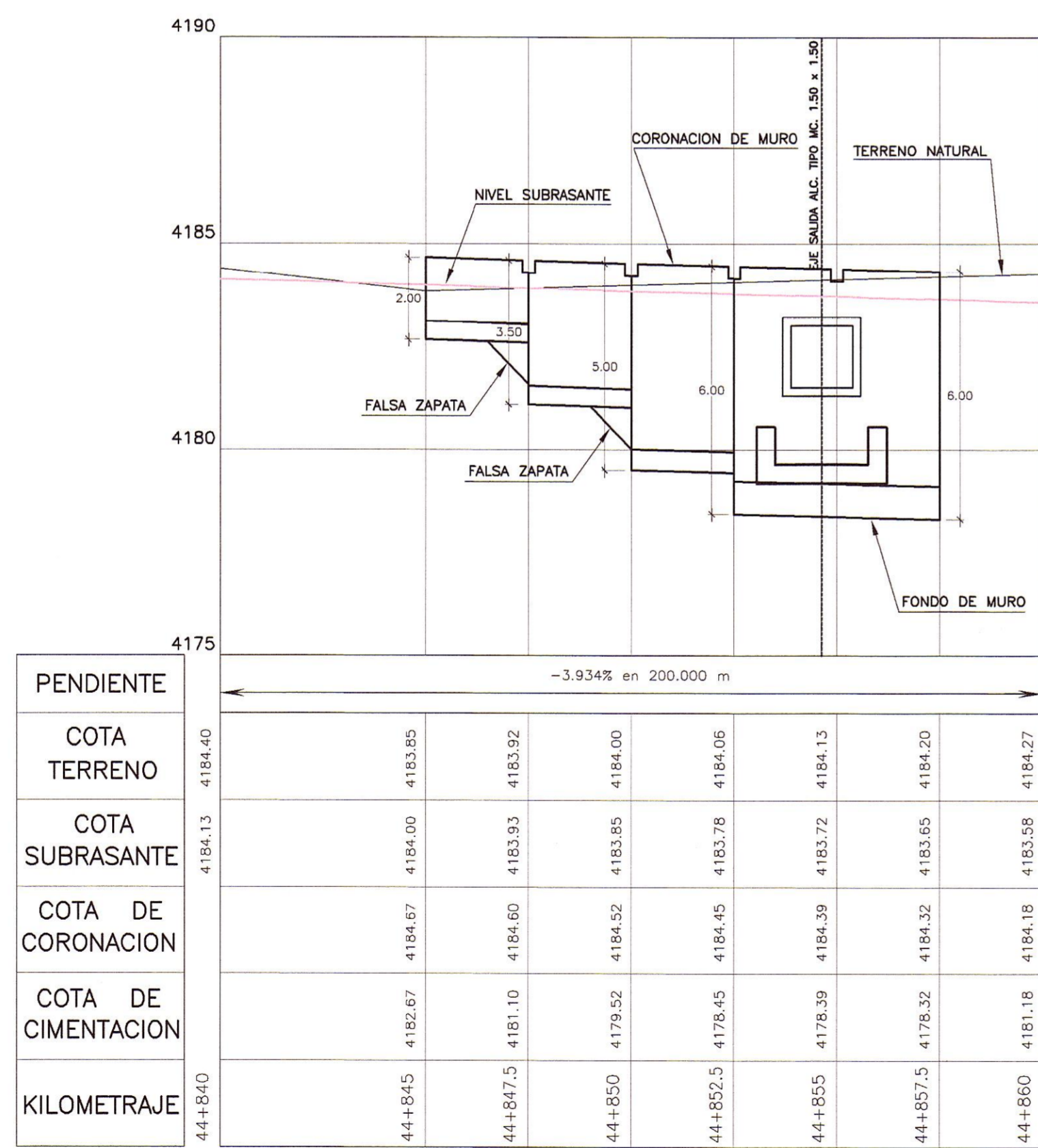
PERFIL LONGITUDINAL ESC.: H=1/125 V=1/125
