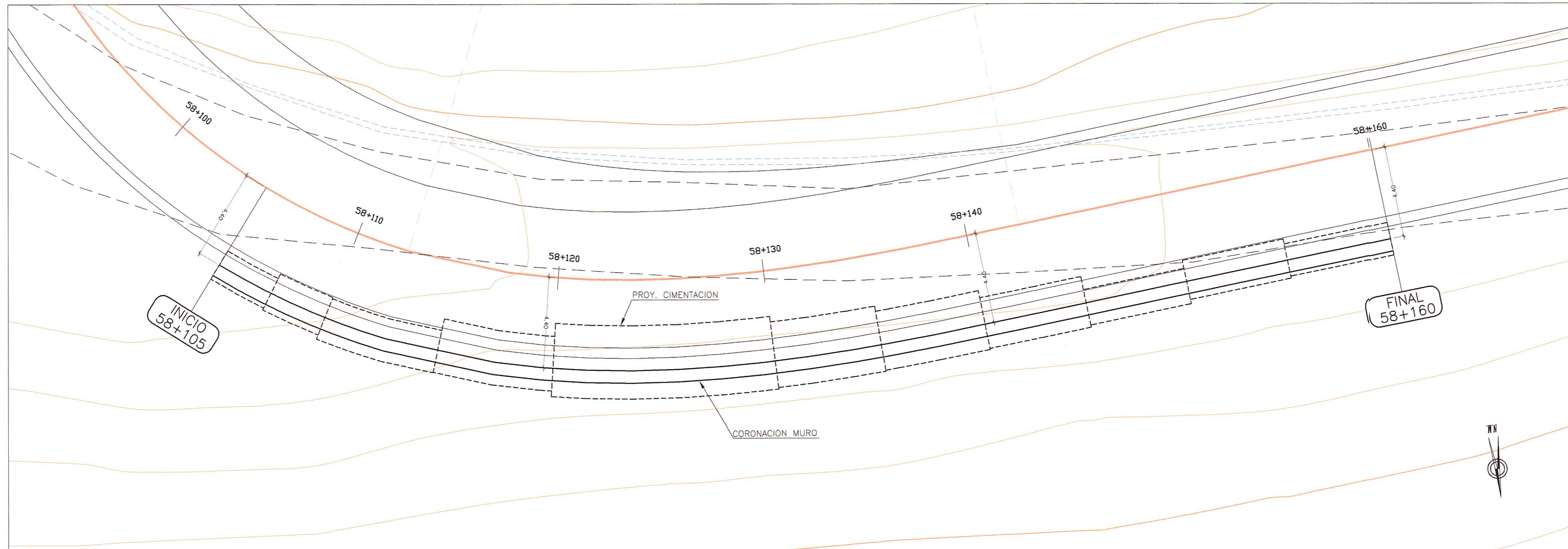
PLANTA ESC. : 1/125
