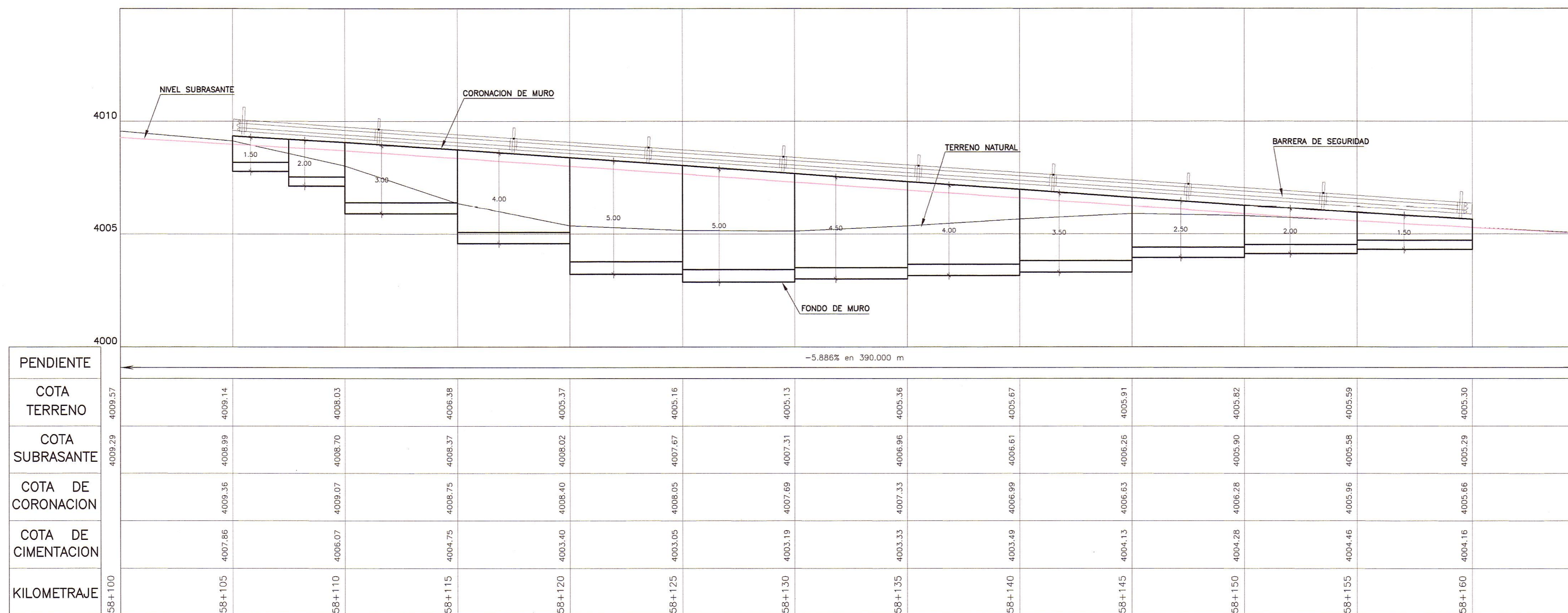
PERFIL LONGITUDINAL ESC. : H=1/125 V=1/125
