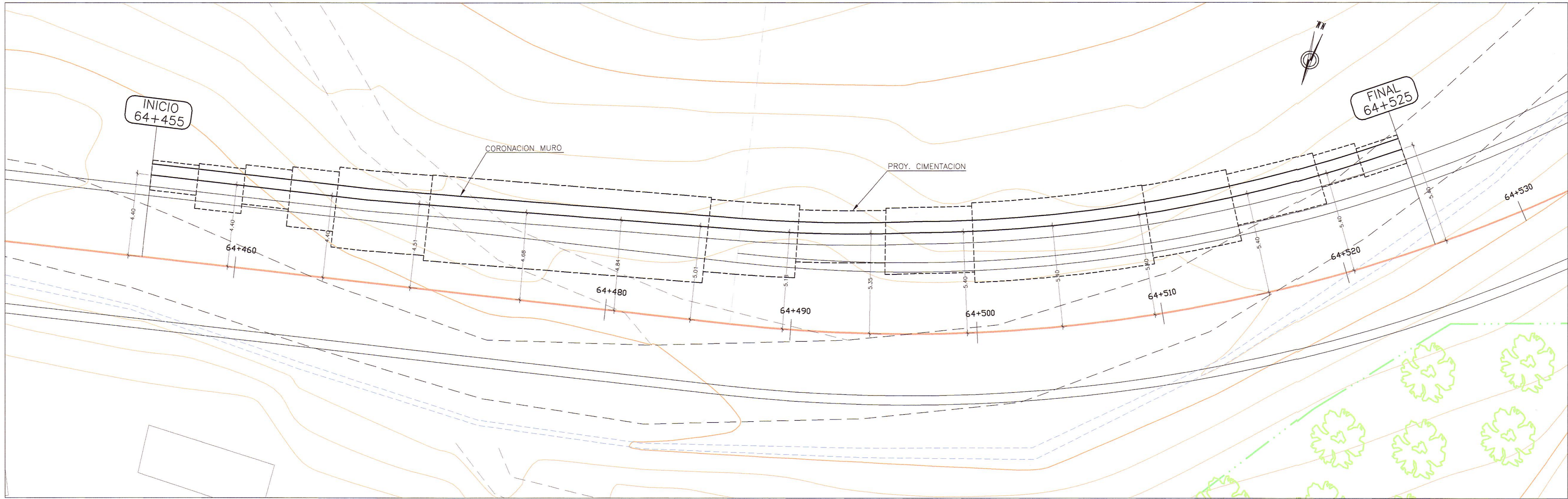
PLANTA ESC. : 1/125
