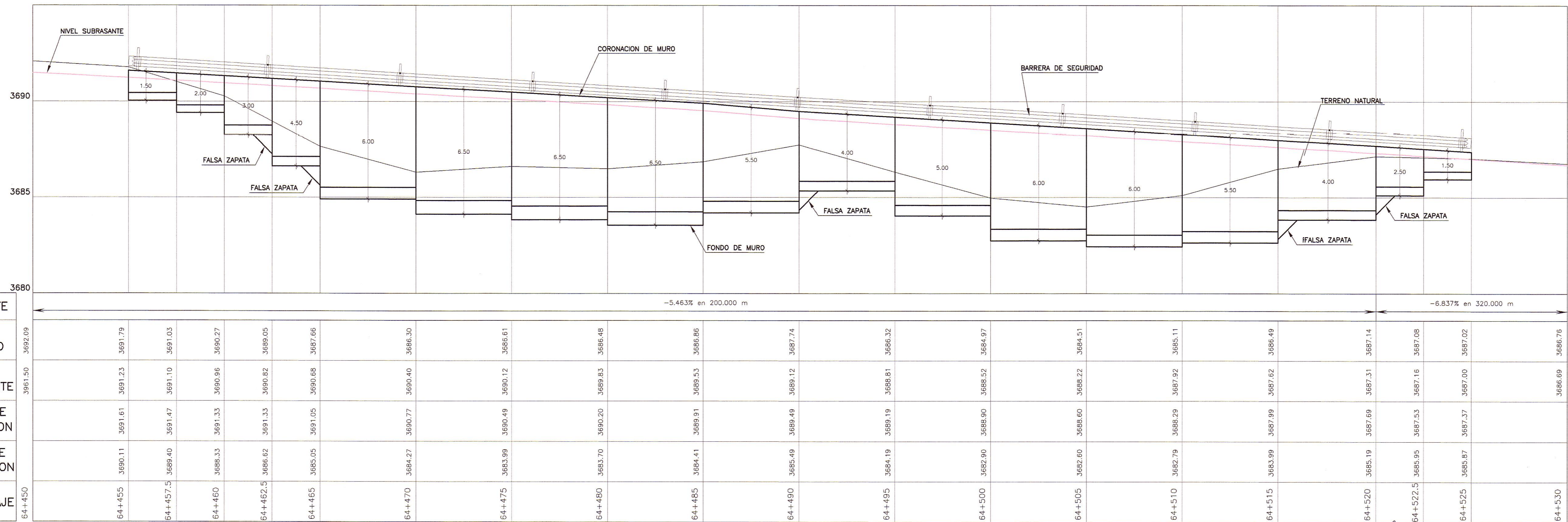
PERFIL LONGITUDINAL
