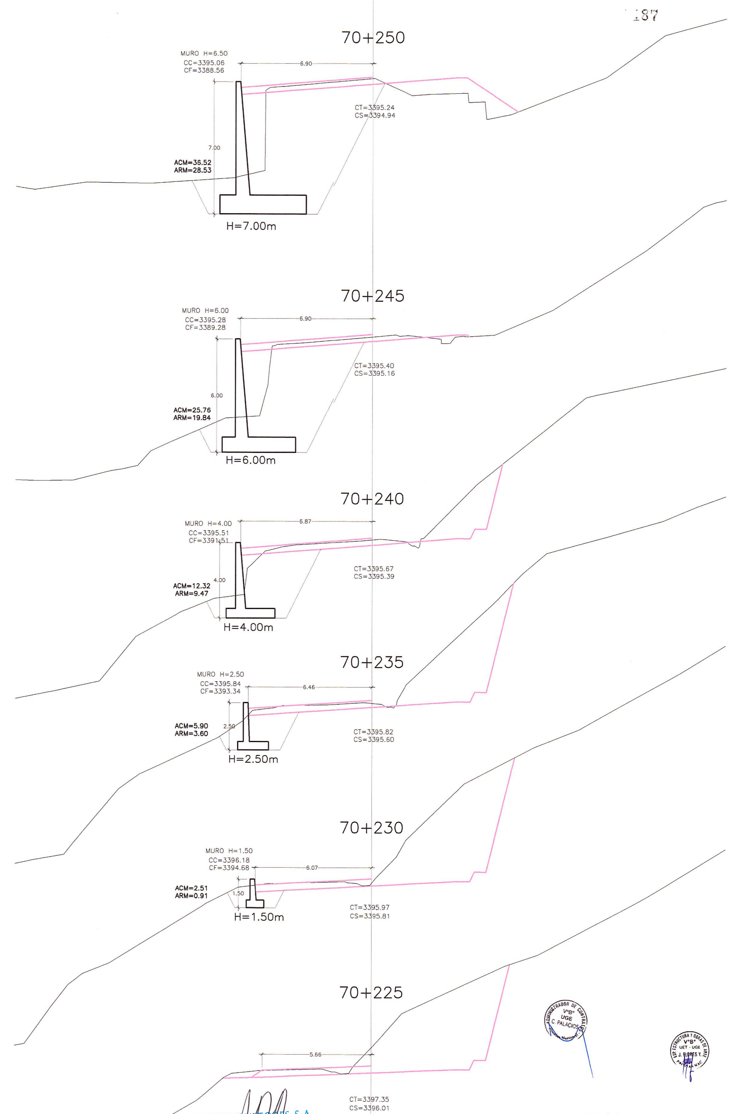
SECCIONES TRANSVERSALES ESC.: 1/125
