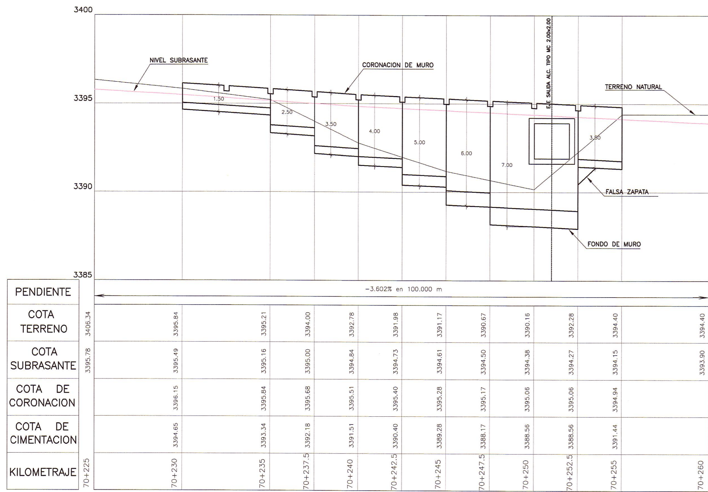
PERFIL LONGITUDINAL
