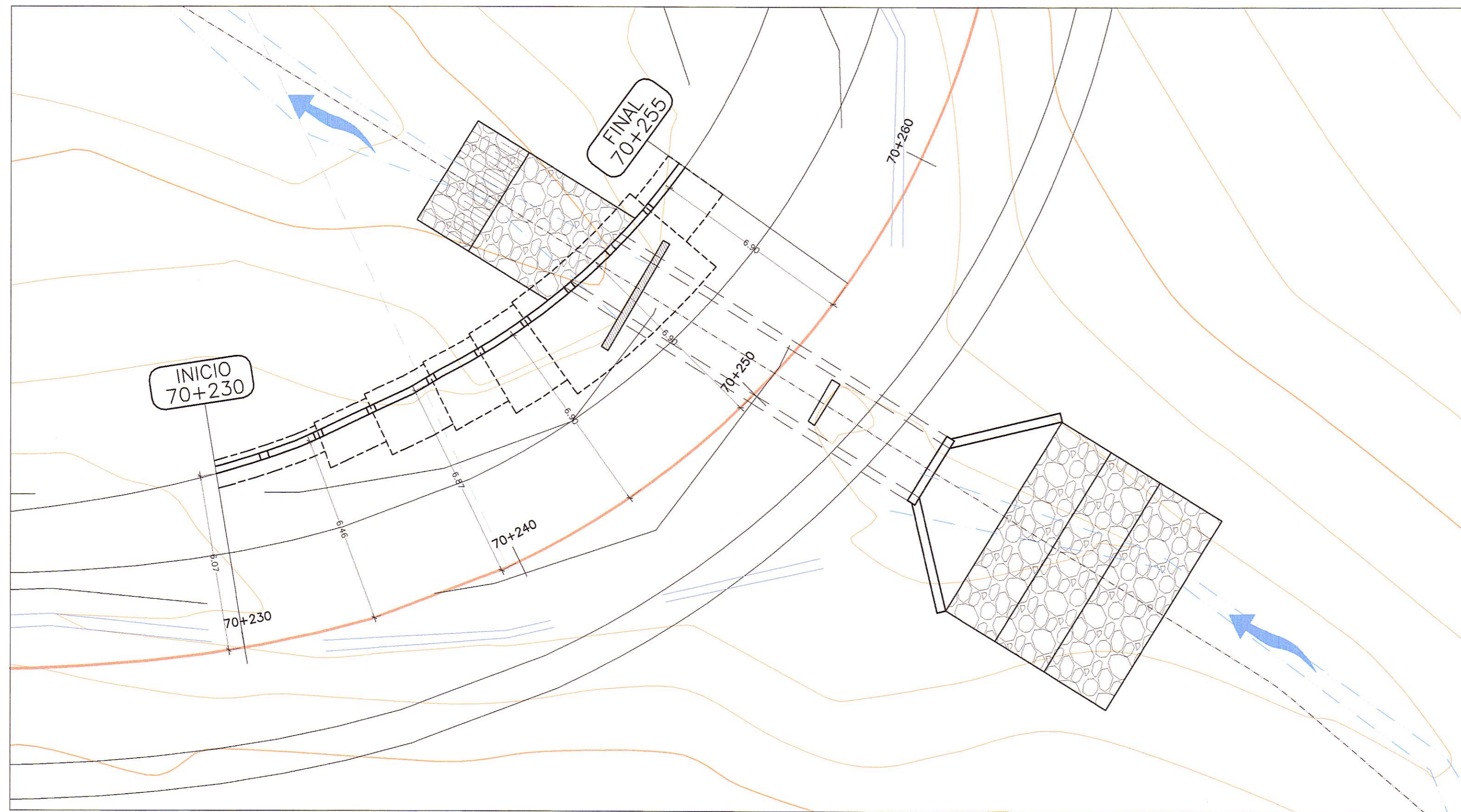
PLANTA ESC.: 1/125
