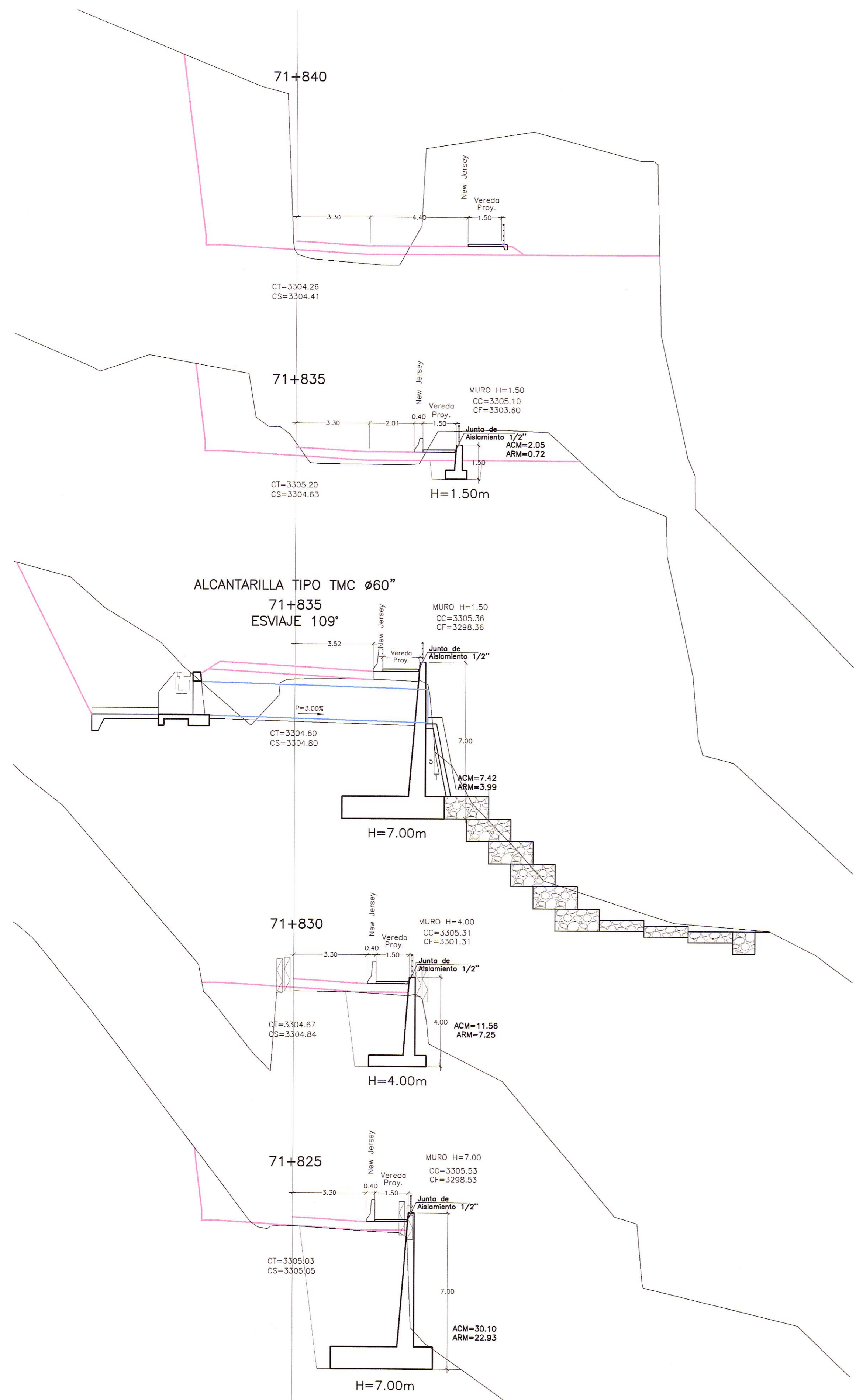
SECCIONES TRANSVERSALES ESC. : 1/125
