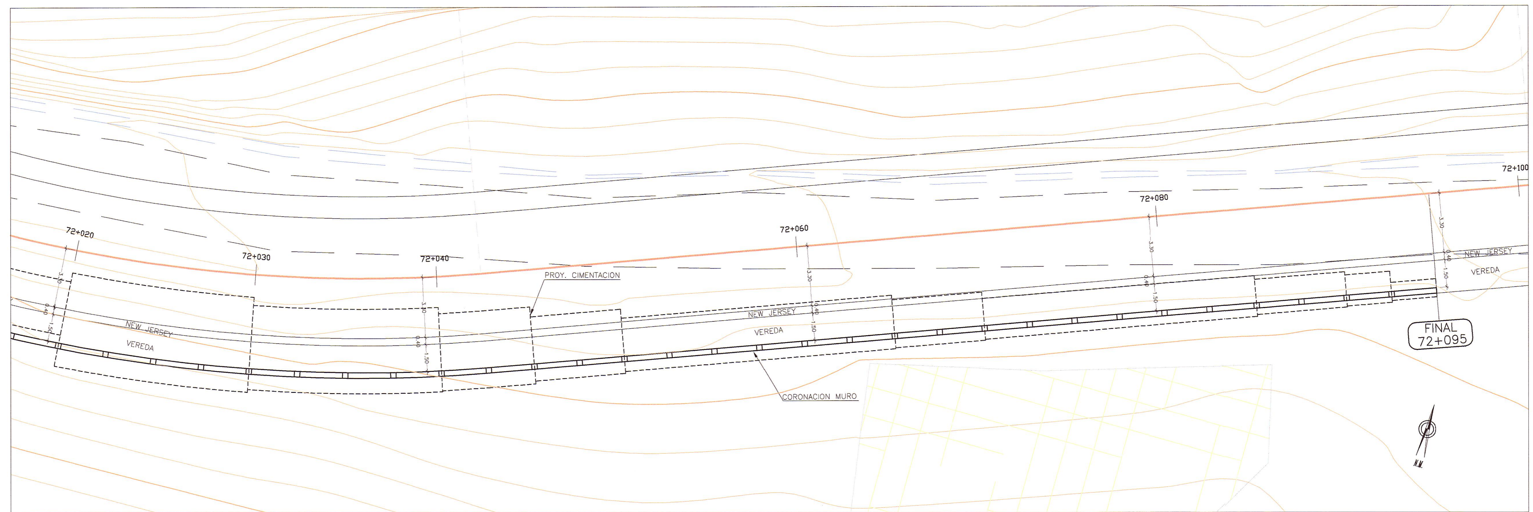
PLANTA ESC. : 1/125
