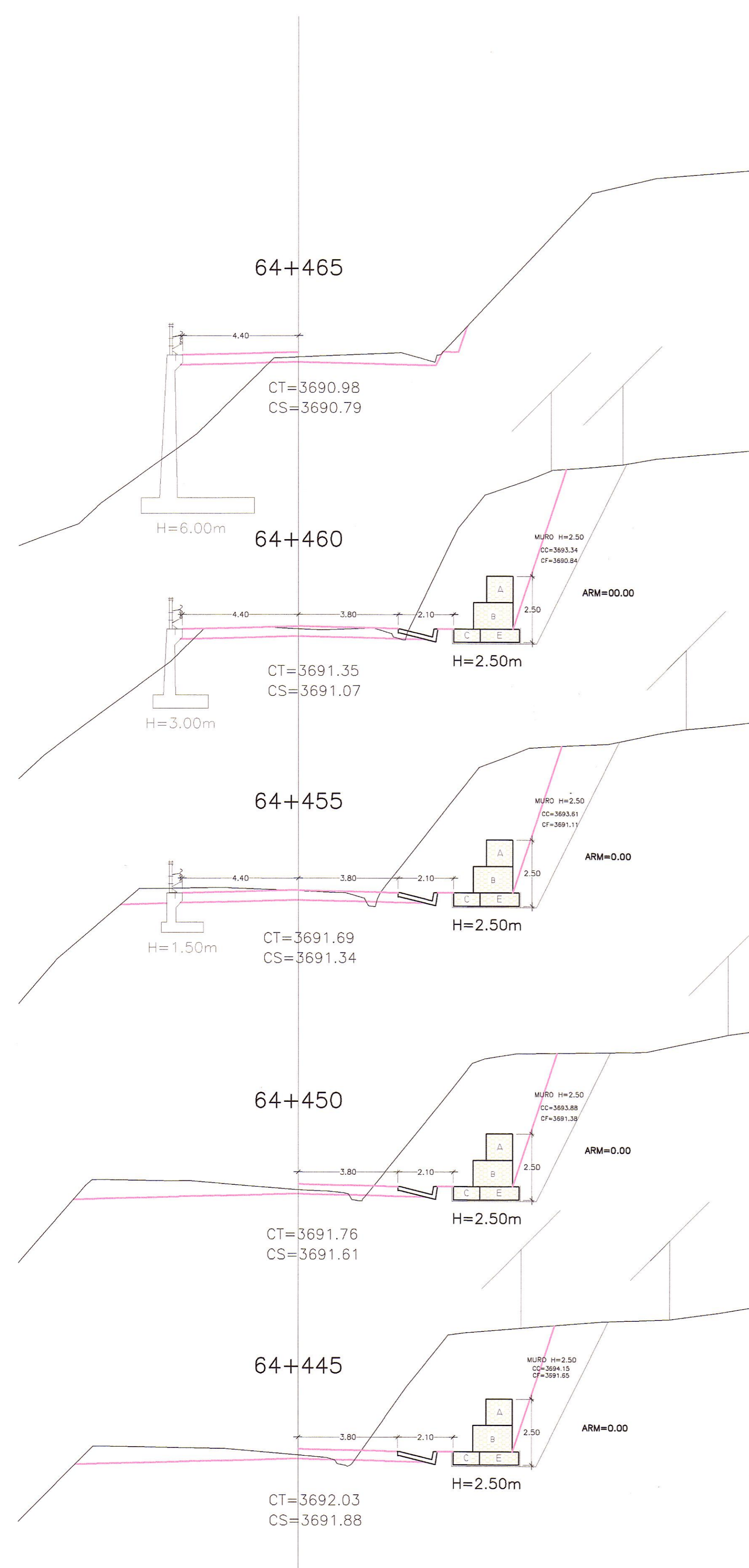
SECCIONES TRANSVERSALES ESC. : 1/125
