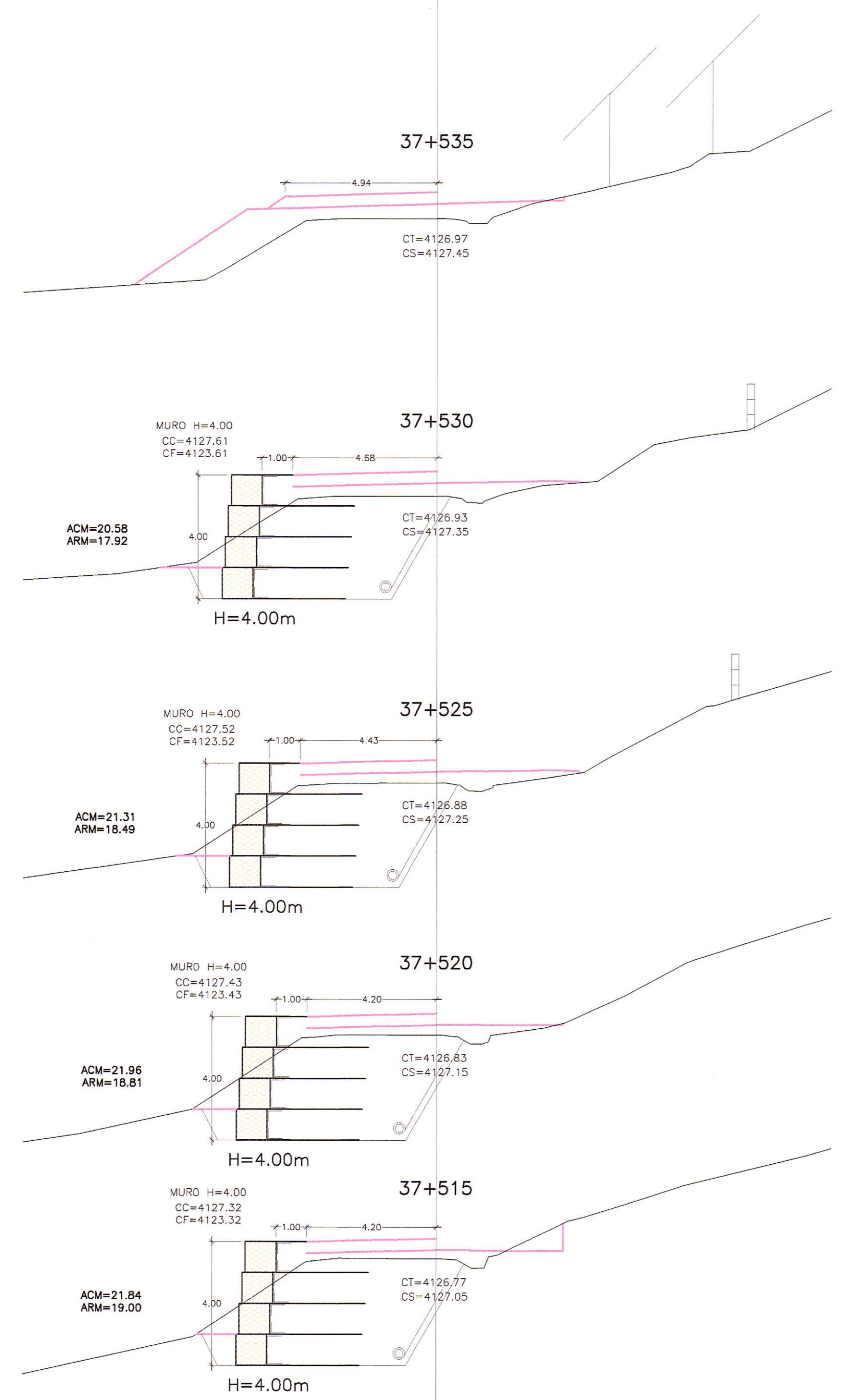
SECCIONES TRANSVERSALES ESC. : 1/125
