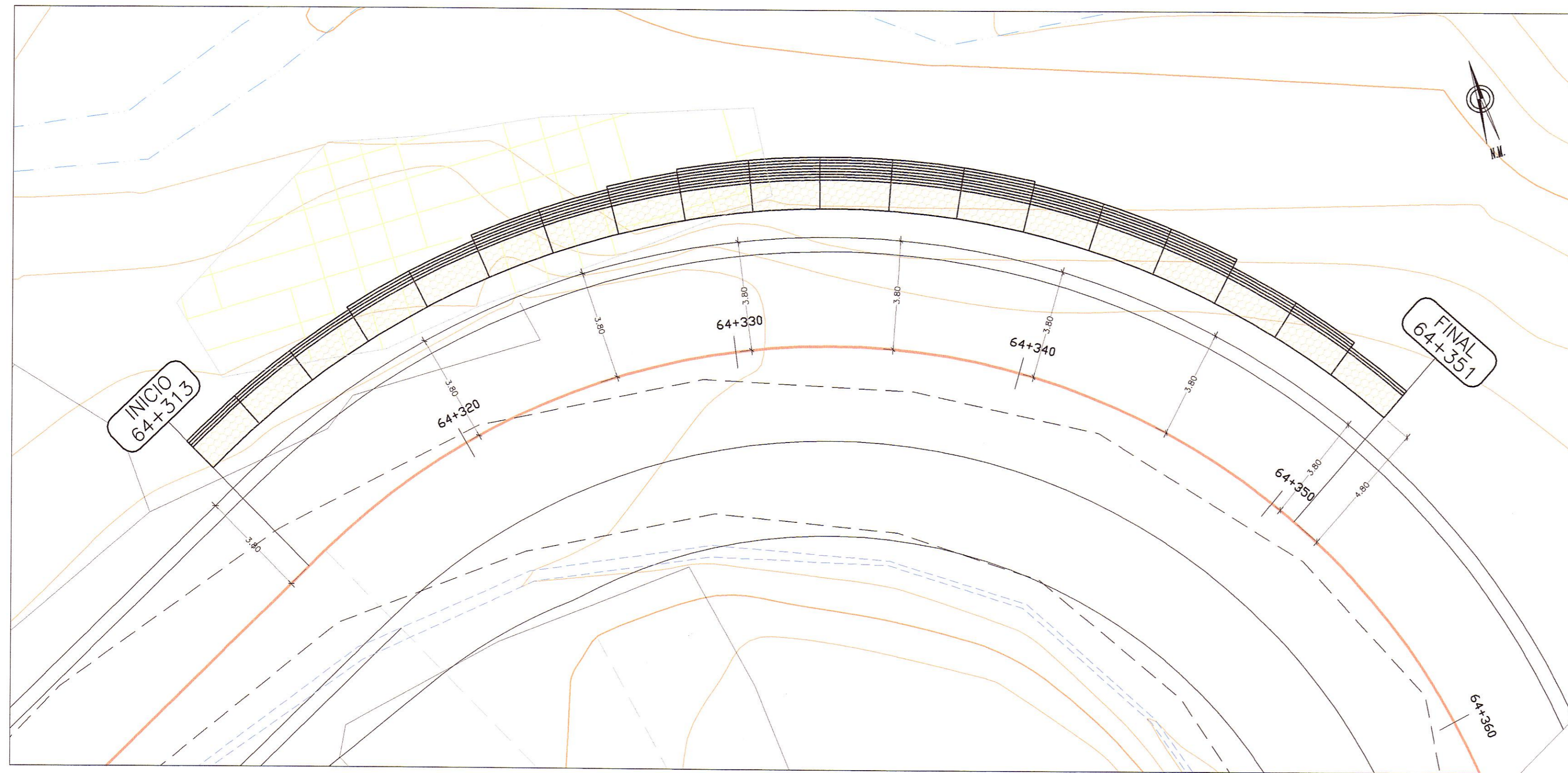
PLANTA ESC. : 1/125
