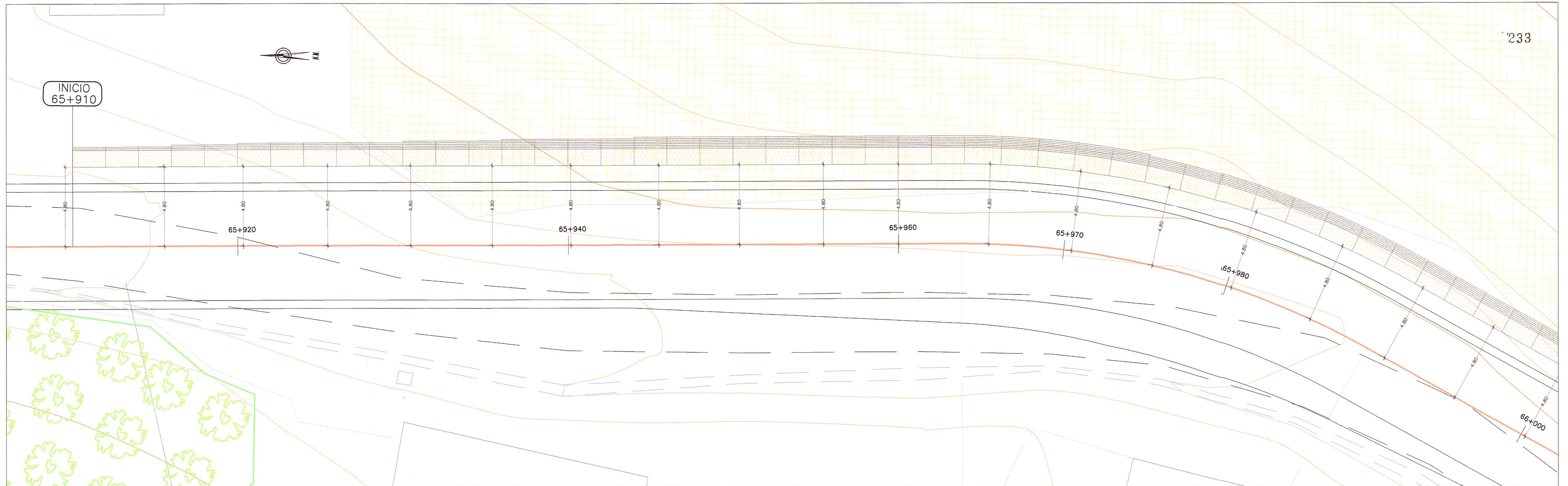
PLANTA ESC. : 1/125
