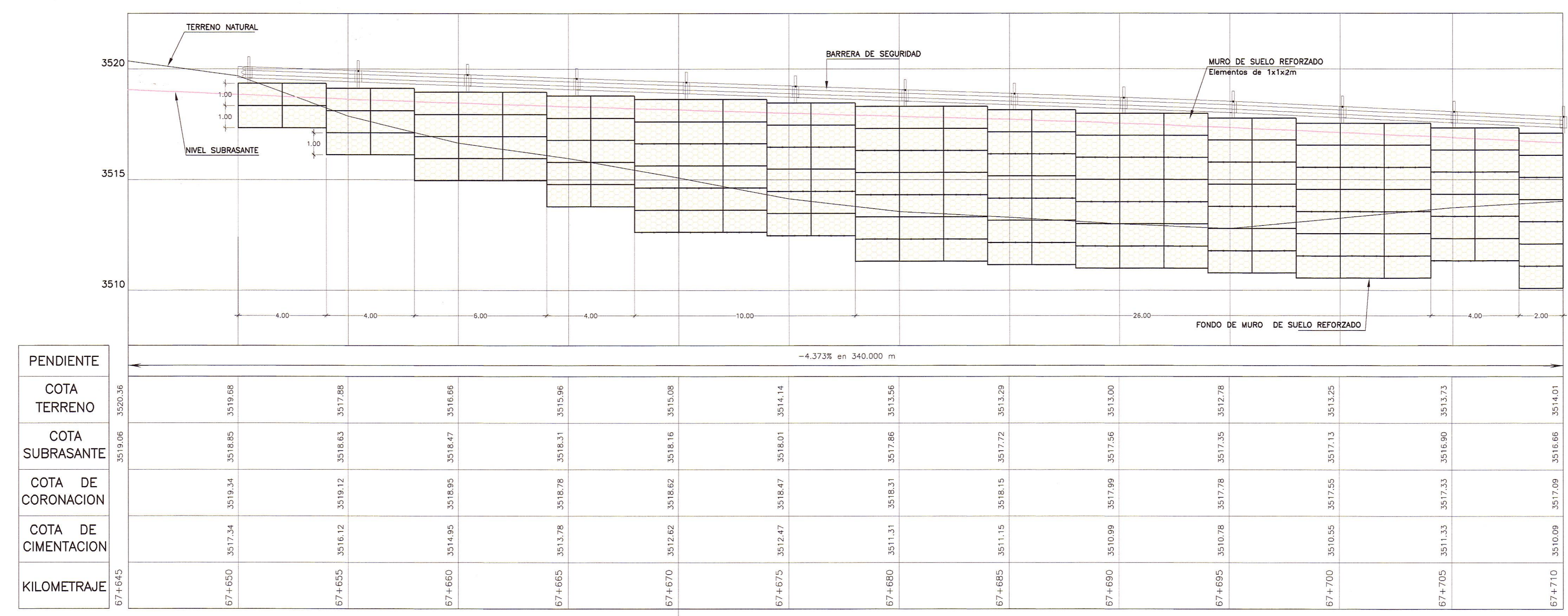
PERFIL LONGITUDINAL ESC. : H=1/125 V=1/125
