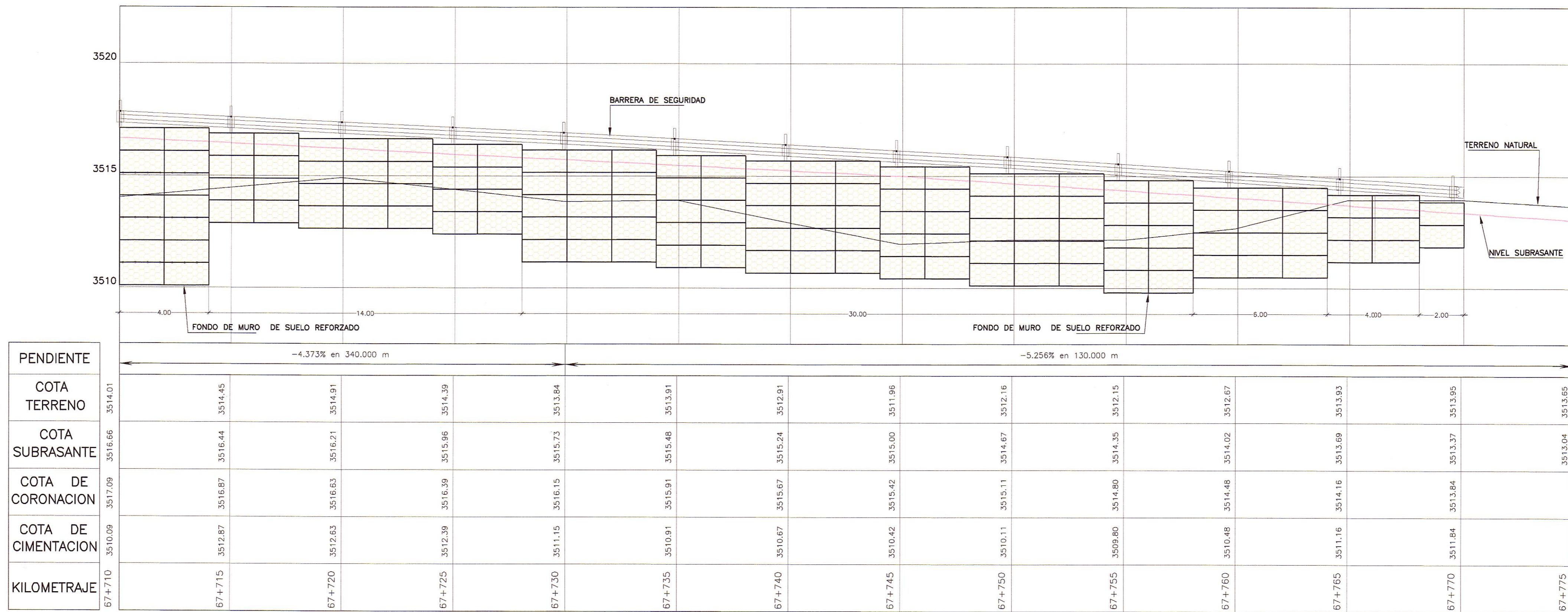
PERFIL LONGITUDINAL
