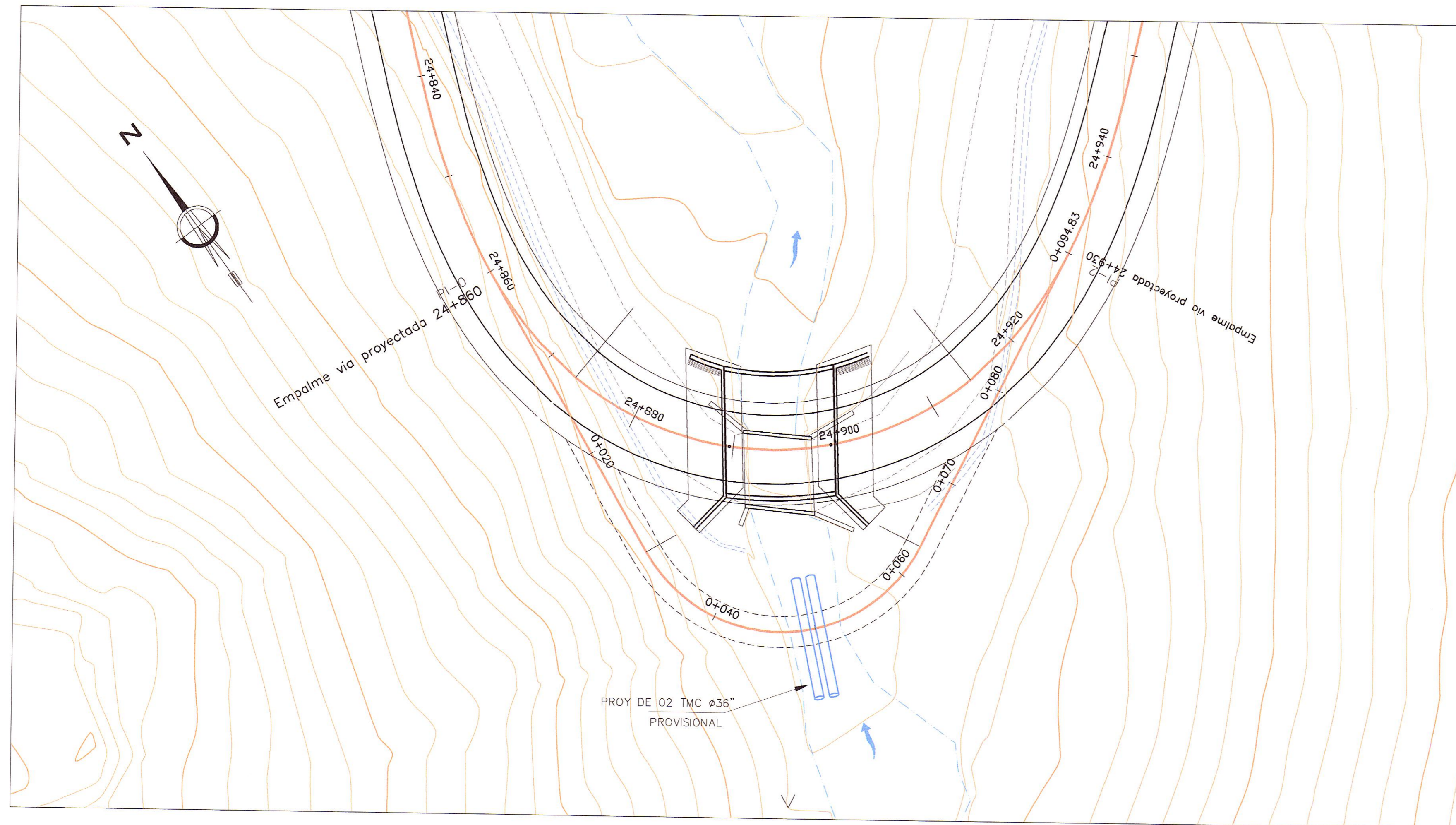
PLANTA 1:300
