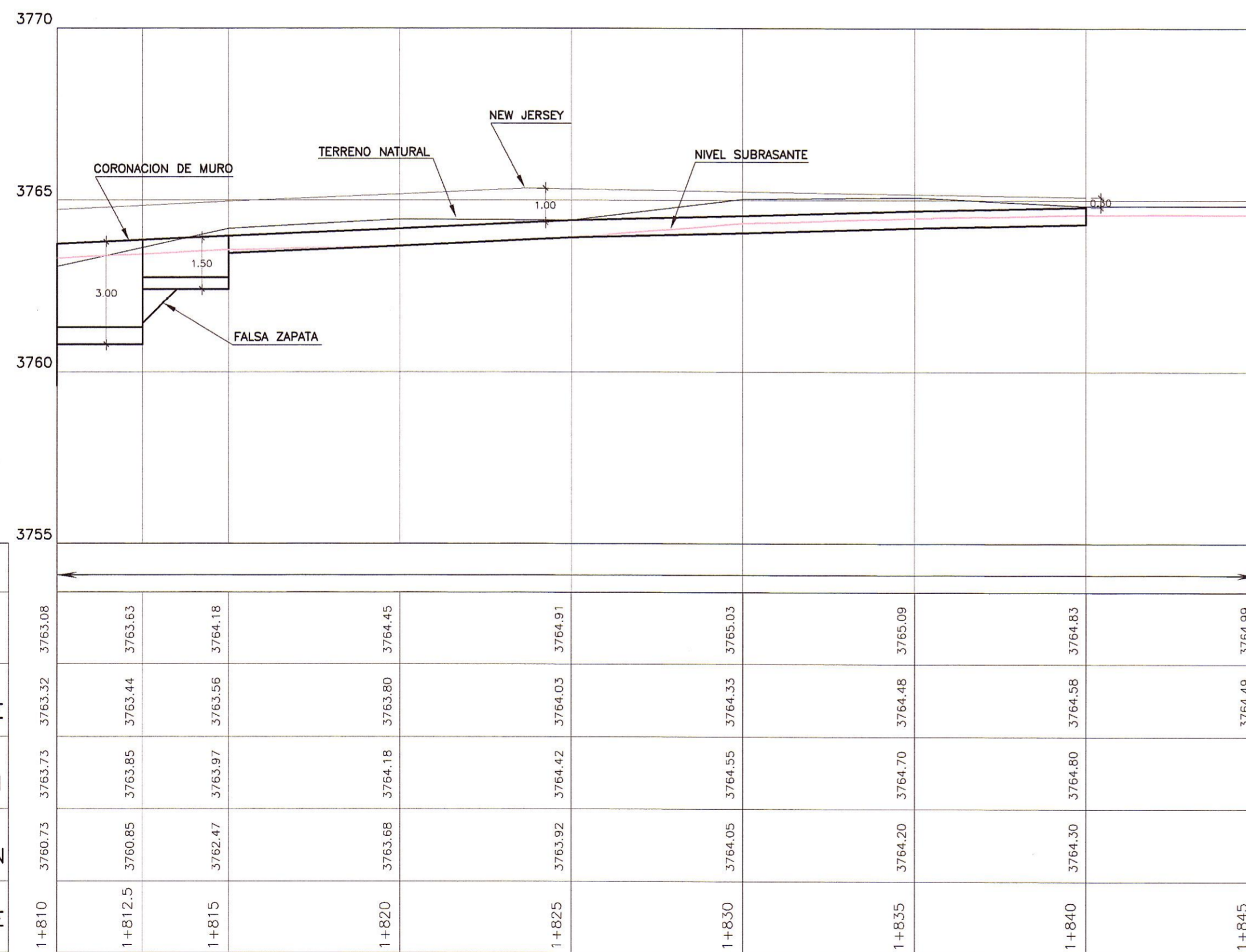
PERFIL LONGITUDINAL
