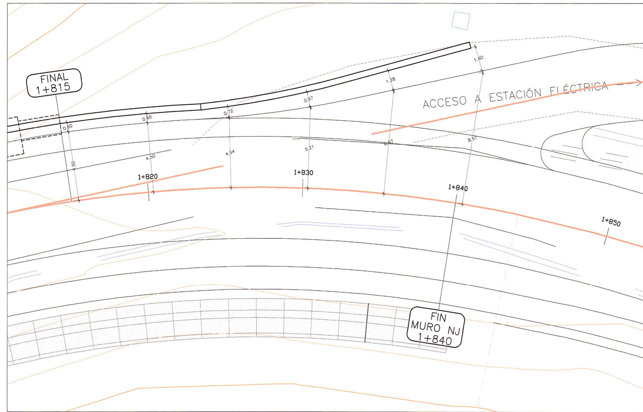
PLANTA ESC. : 1/125
