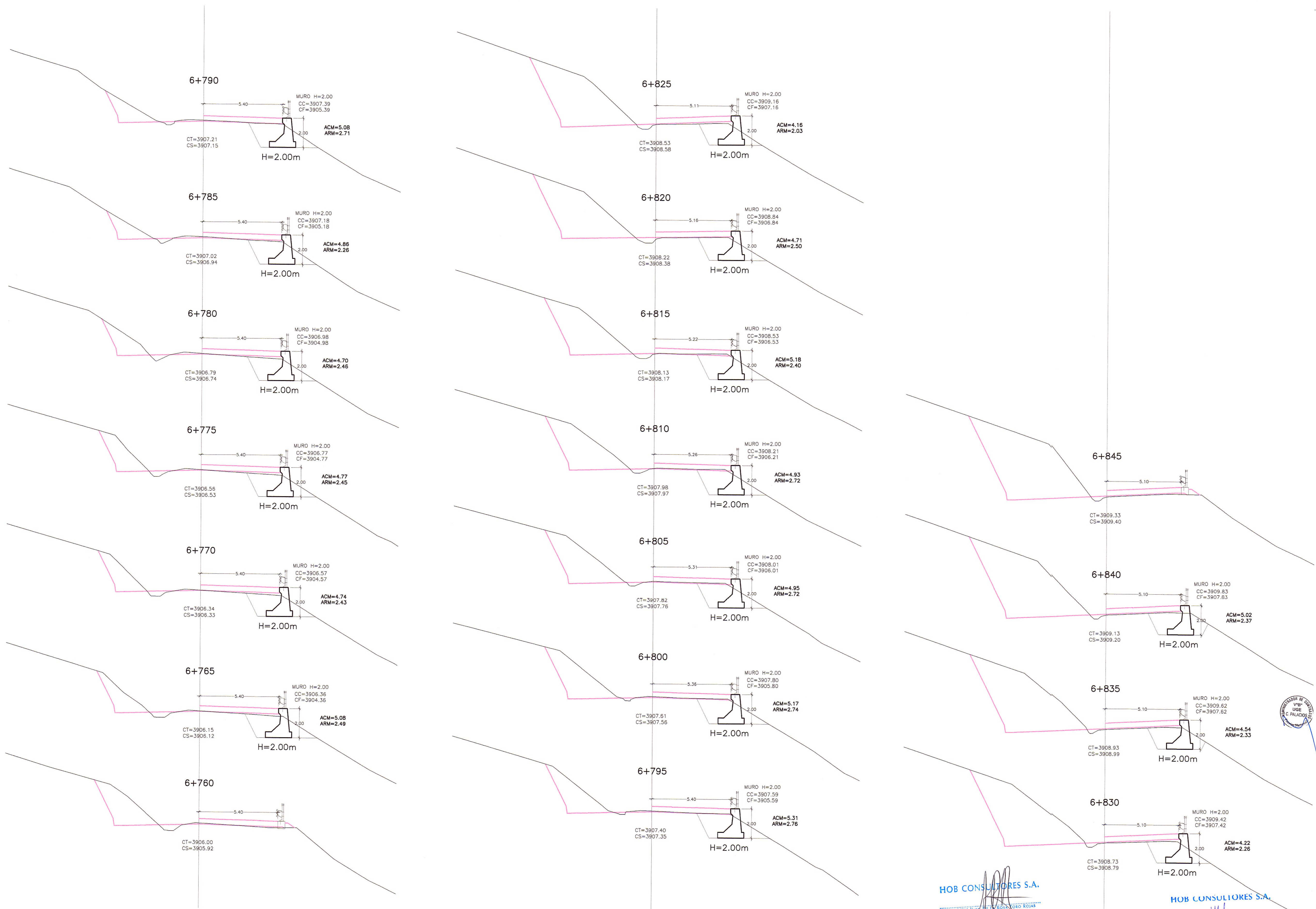
SECCIONES TRANSVERSALES ESC.: 1/125
