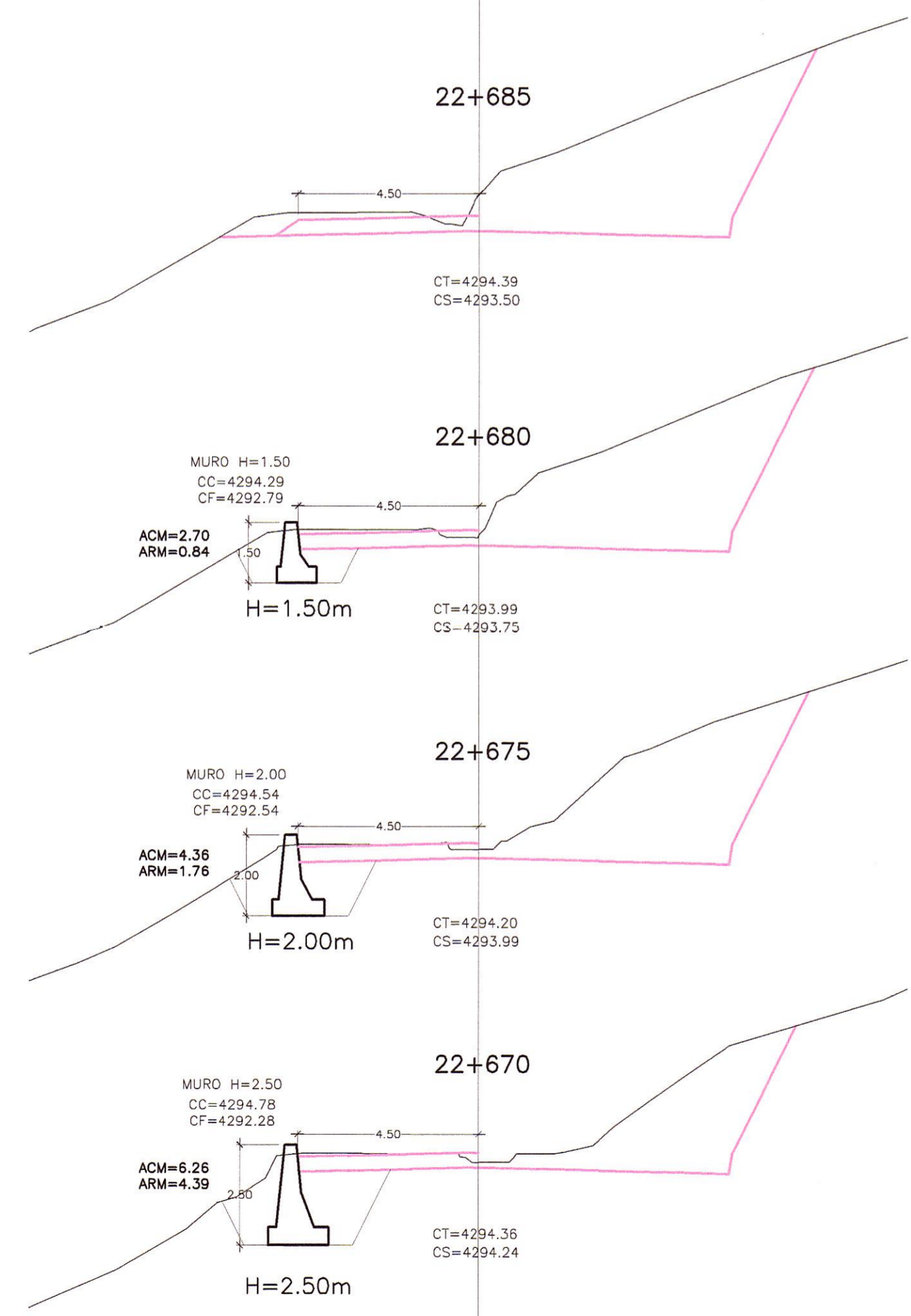
SECCIONES TRANSVERSALES ESC. 1: 1/125
