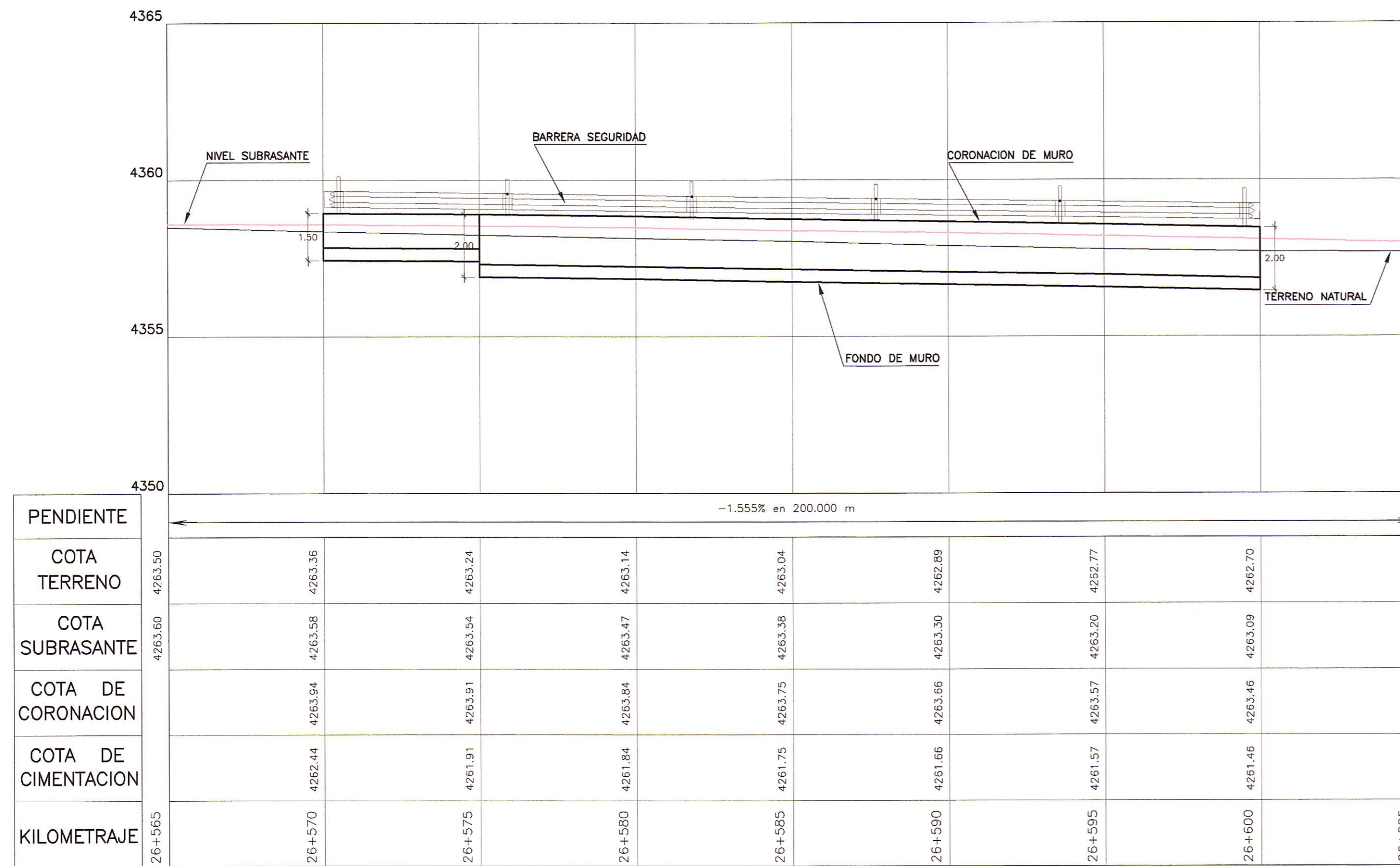
PERFIL LONGITUDINAL
