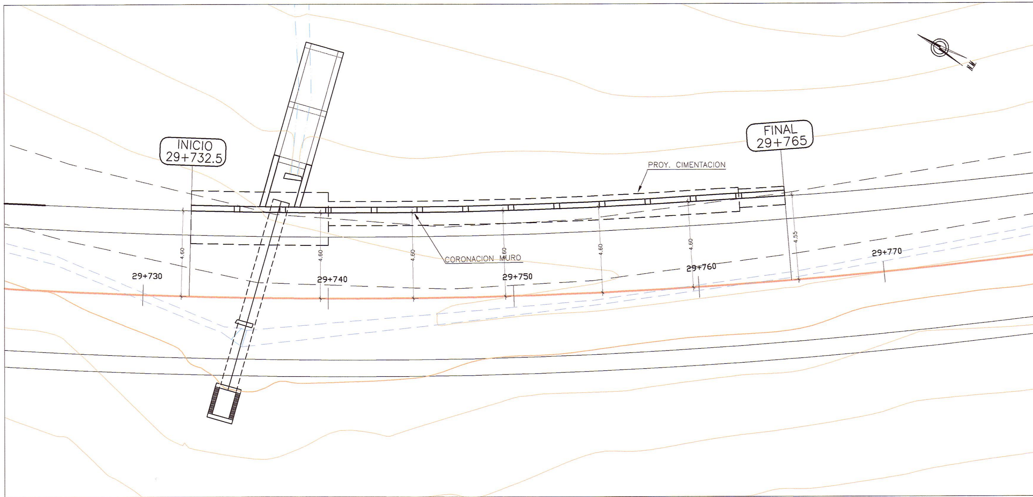
PLANTA ESC. : 1/125
