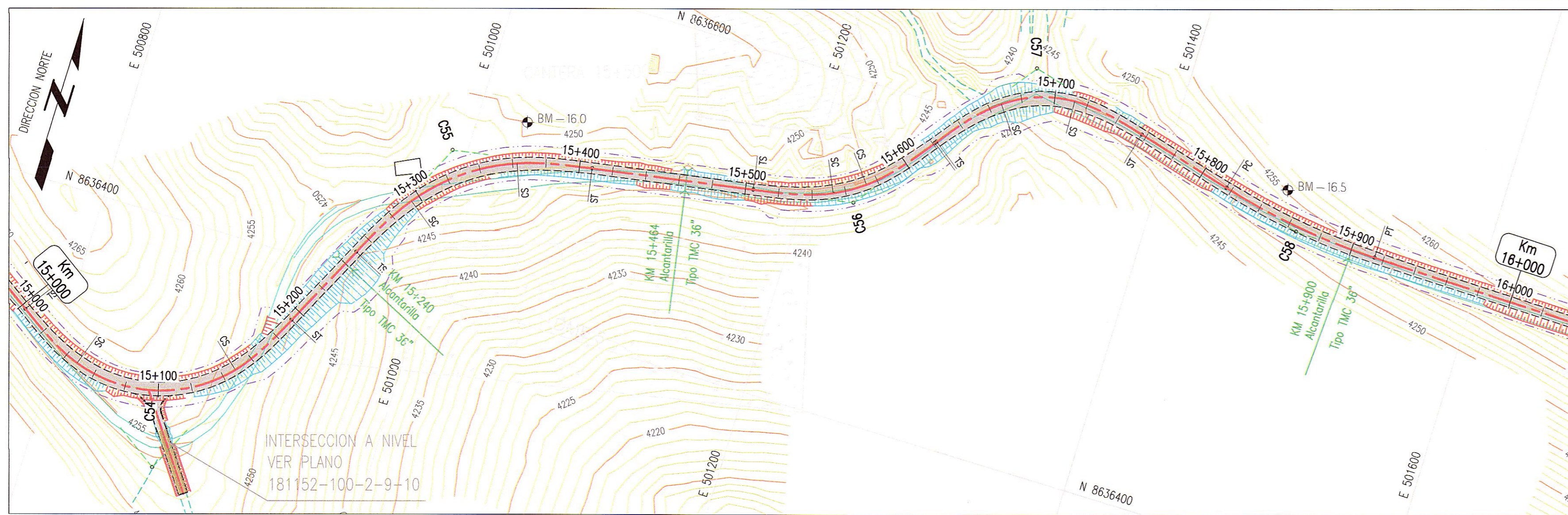
PLANTA ESC 1:2000
