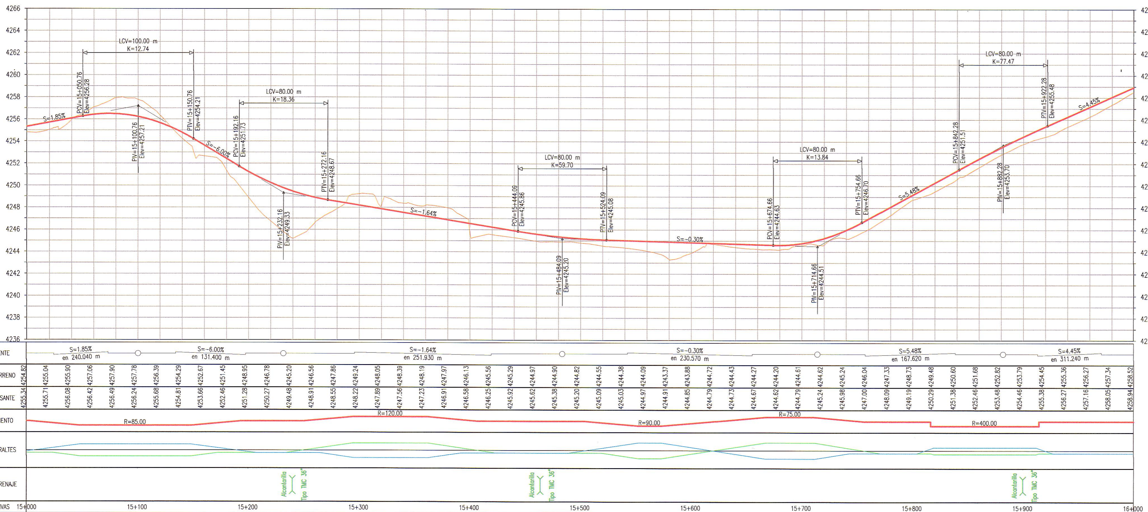
PERFIL LONGITUDINAL ESC H 1:2000 V 1:200
