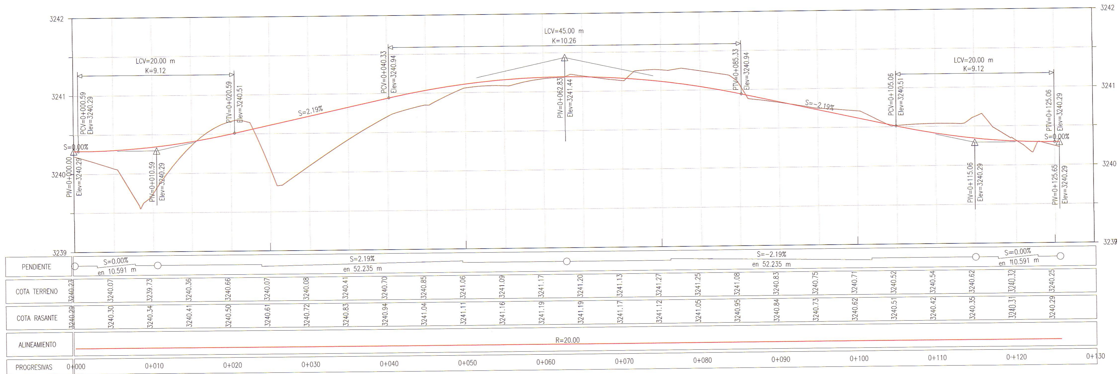
PERFIL LONGITUDINAL - OVALO H=1:250, V=1:25
