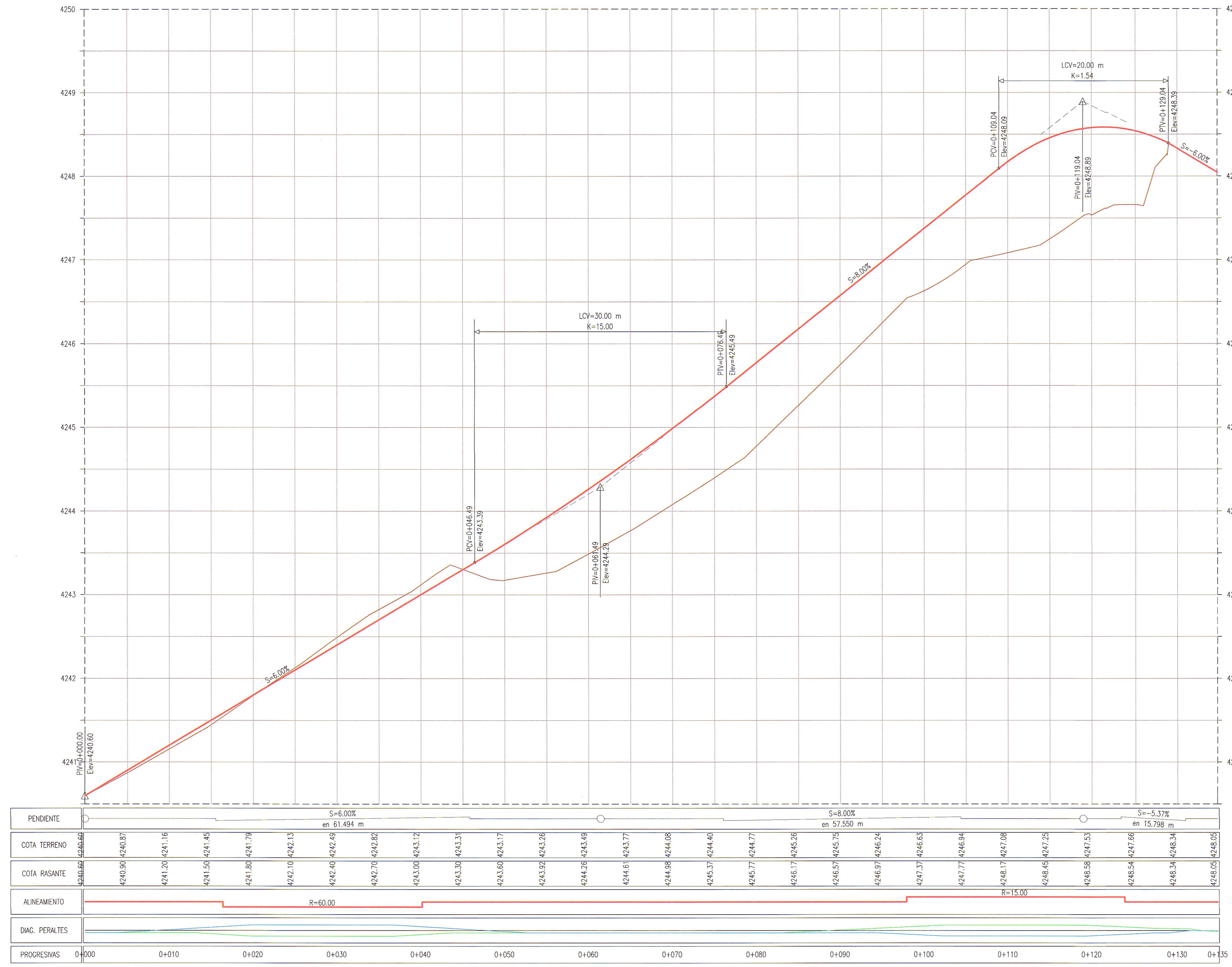
PERFIL LONGITUDINAL IZQUIERDO (INTERSECCIÓN TIPO "T" 14+670) ESC H 1:250 V 1:25
