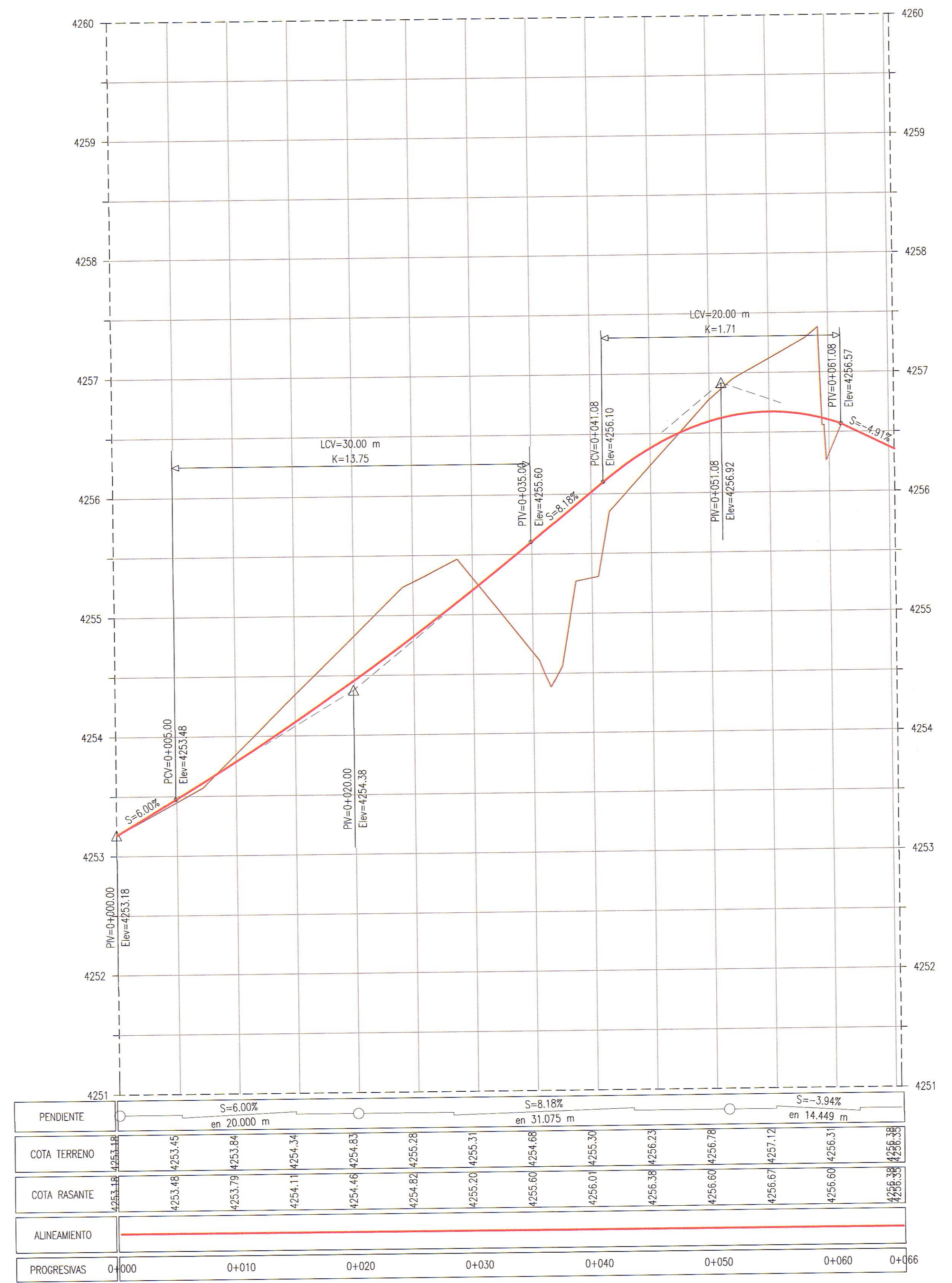
PERFIL LONGITUDINAL (INTERSECCIÓN TIPO "T" 15+100) ESC H 1:500 V 1:50
