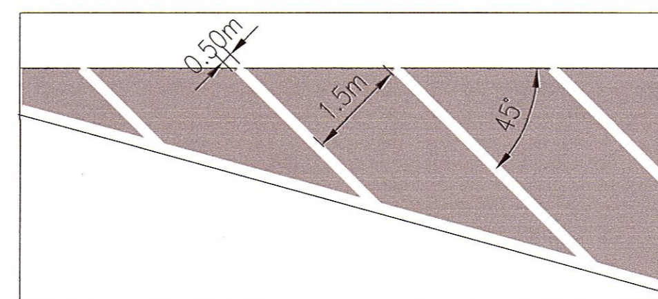
DETALLE 01 CUÑA DE TRANSICION
