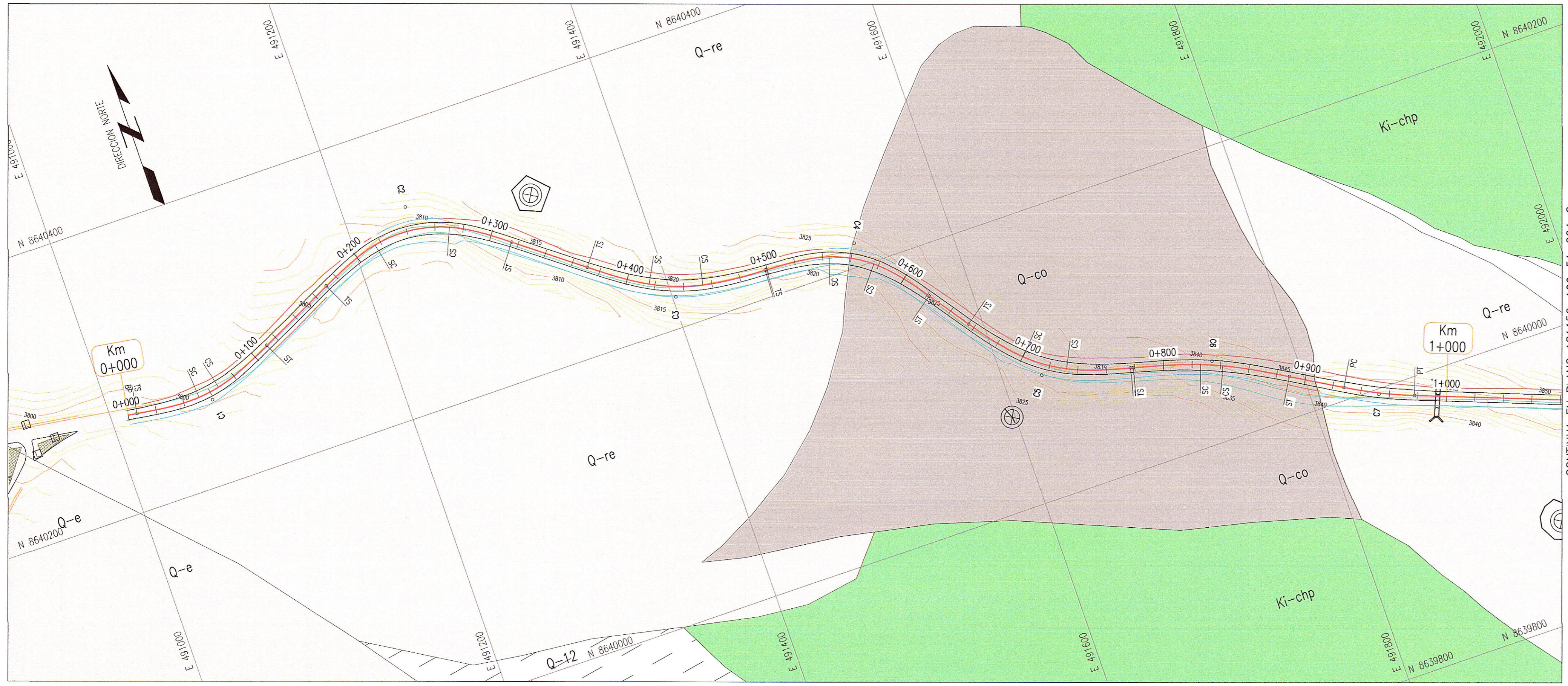
PLANTA 1:2000
