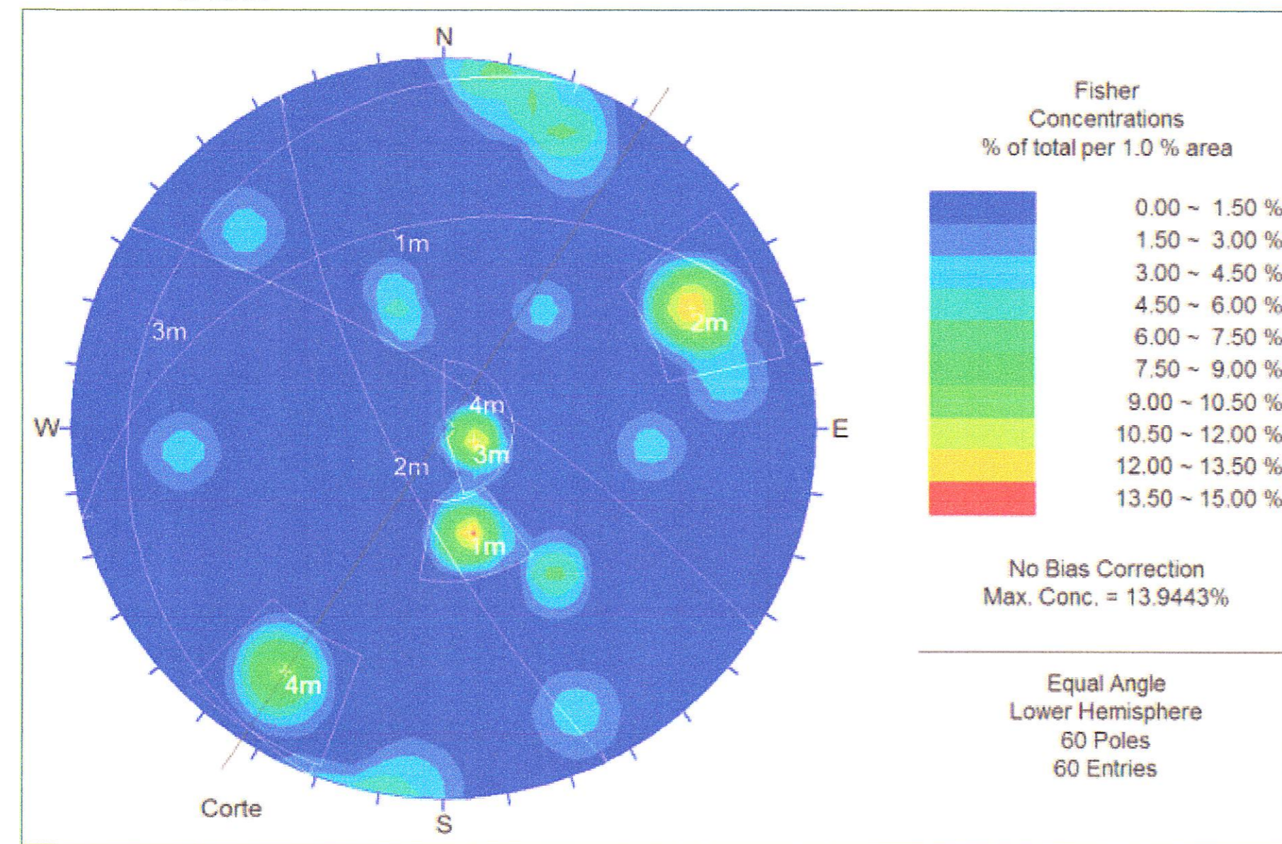
ESTACION GEOMECANICA N° 6 KM 12+478
