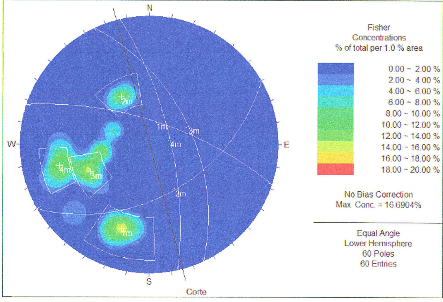
ESTACION GEOMECANICA N° 17 KM 22+525
