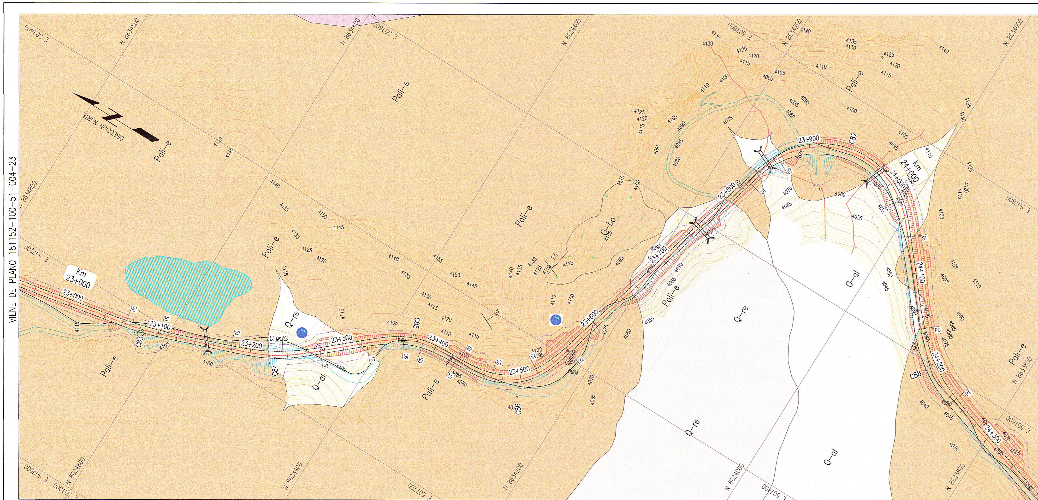
PLANTA 1:2000
