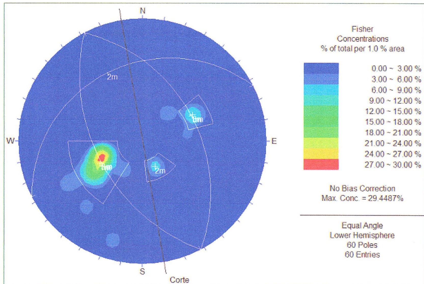
ESTACION GEOMECANICA N° 18 KM 23+260
