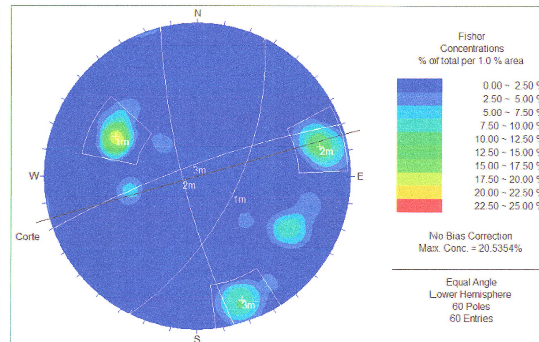
ESTACION GEOMECANICA N° 19 KM 23+570
