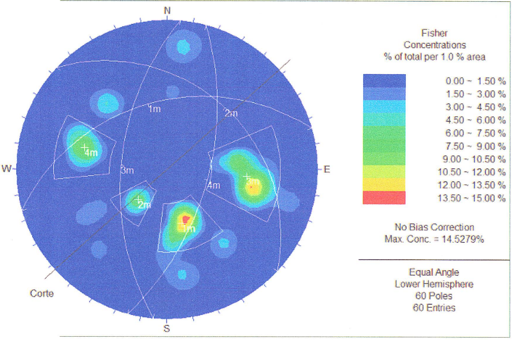
ESTACION GEOMECANICA N° 20 KM 24+080
