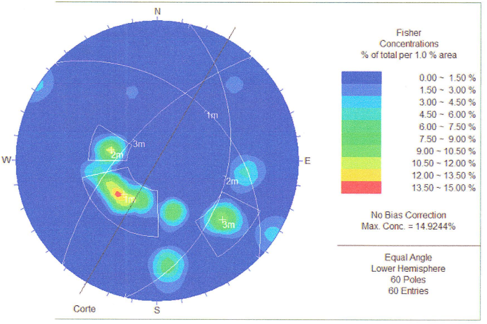
ESTACION GEOMECANICA N° 23 KM 24+490
