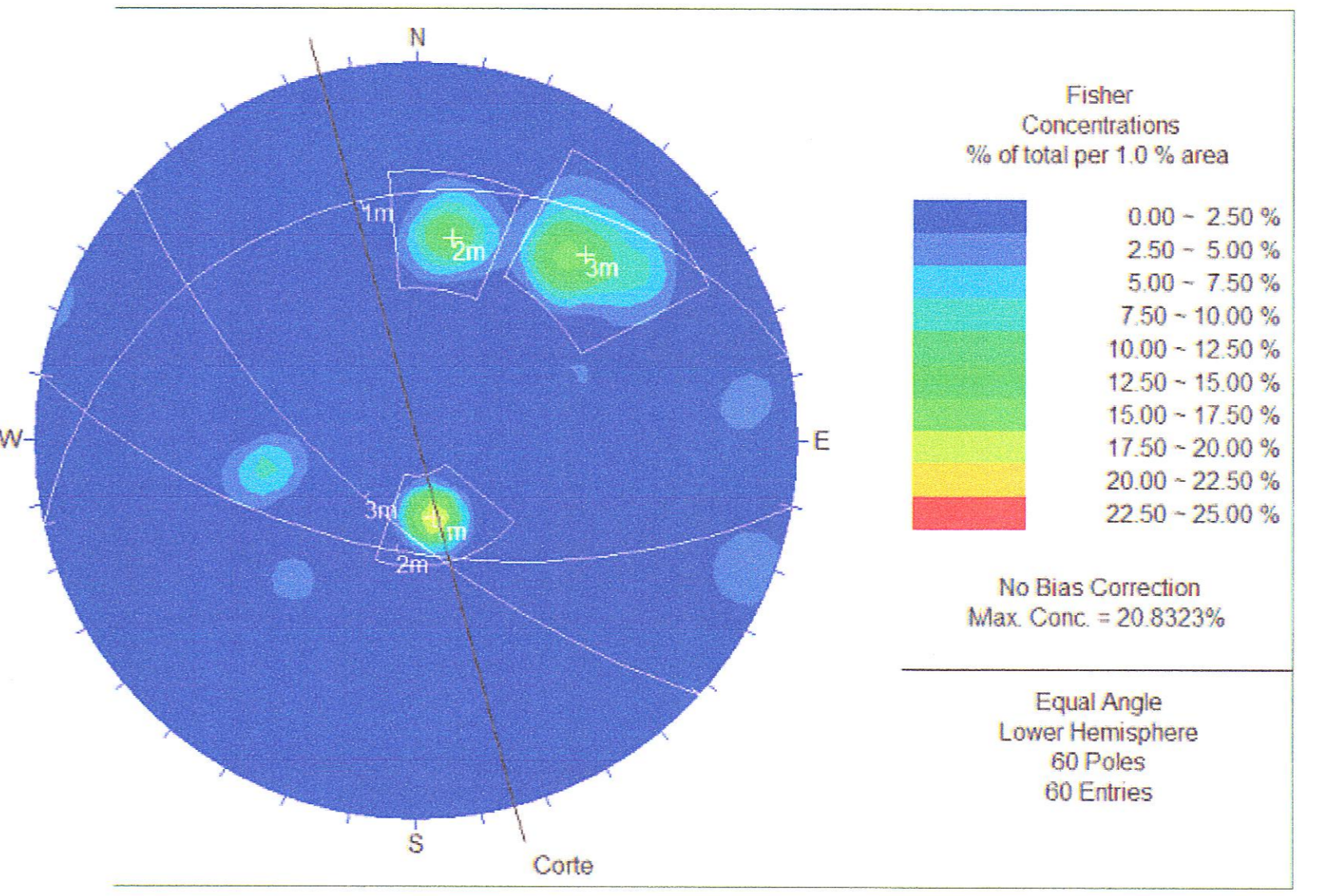
ESTACION GEOMECANICA N° 24 KM 24+740
