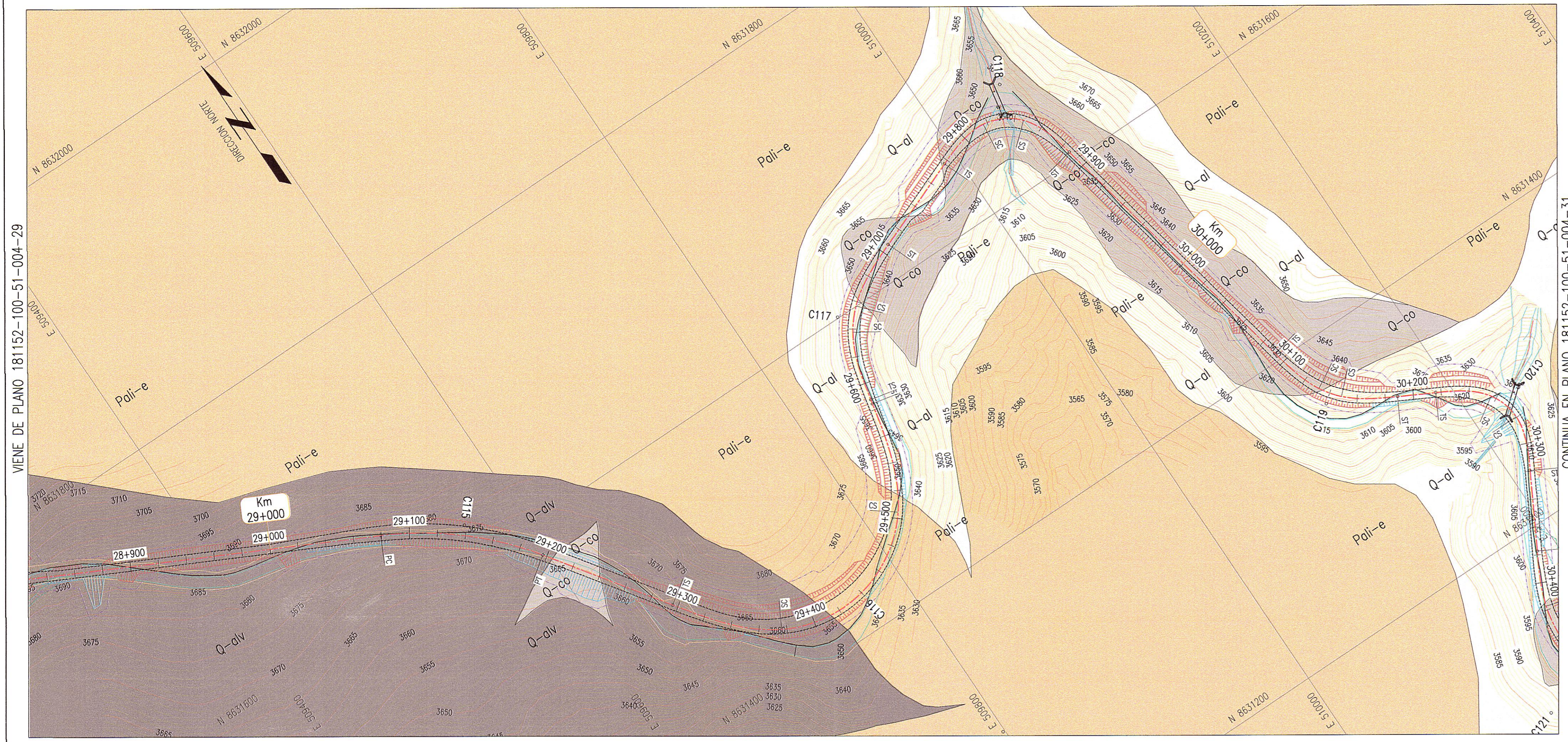
PLANTA 1:2000
