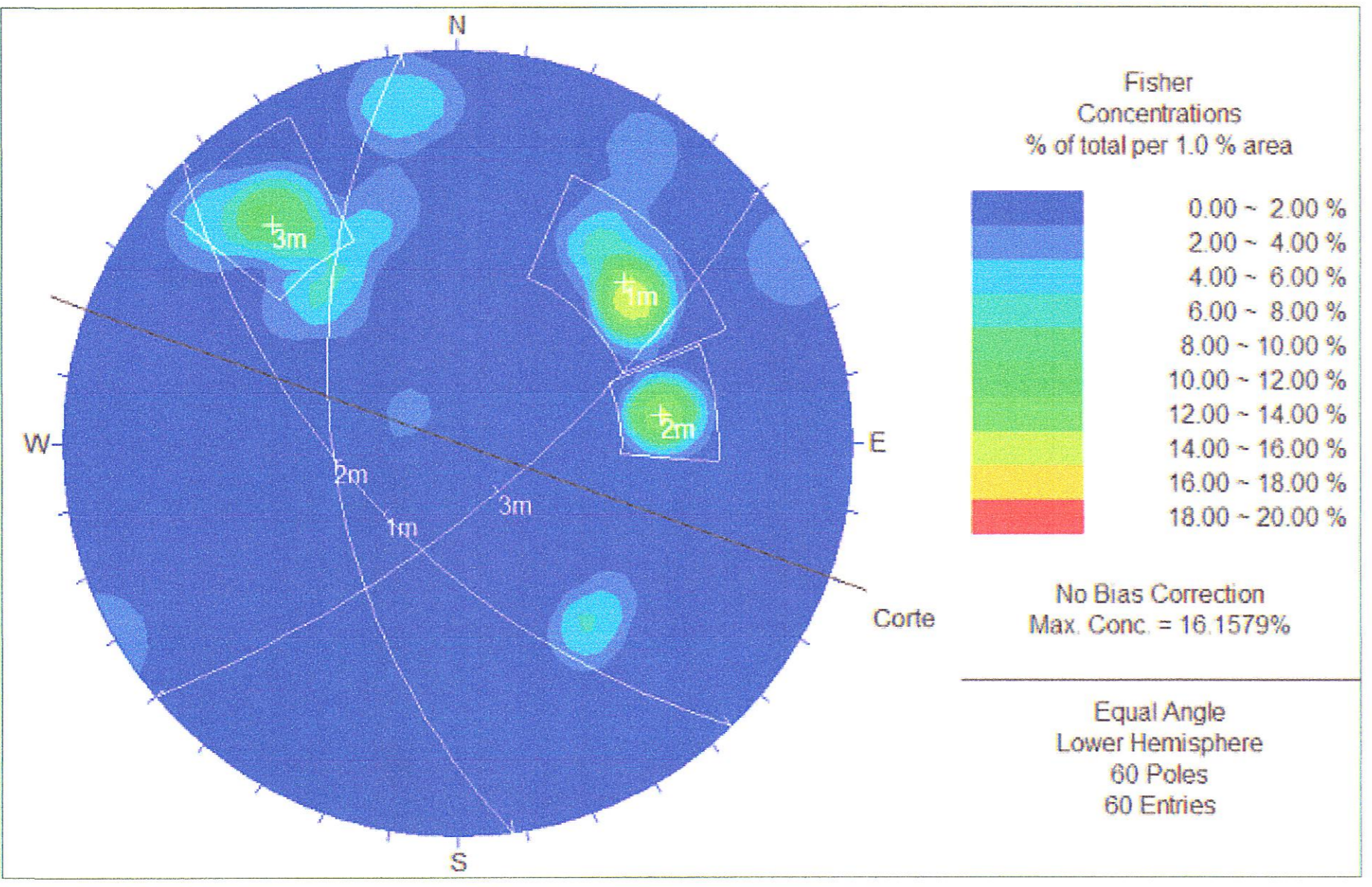
ESTACION GEOMECANICA N° 27 KM 30+610
