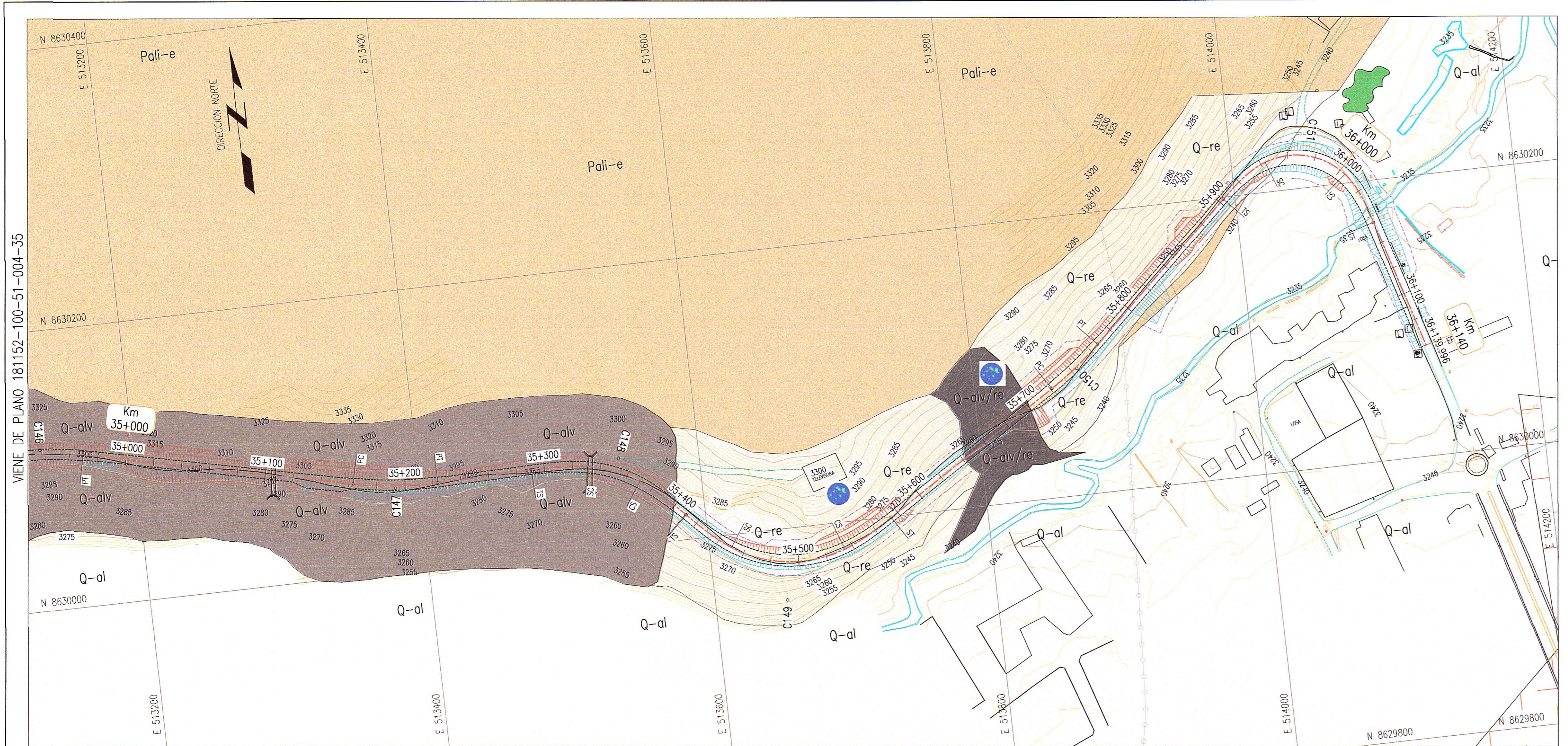
PLANTA 1:2000
