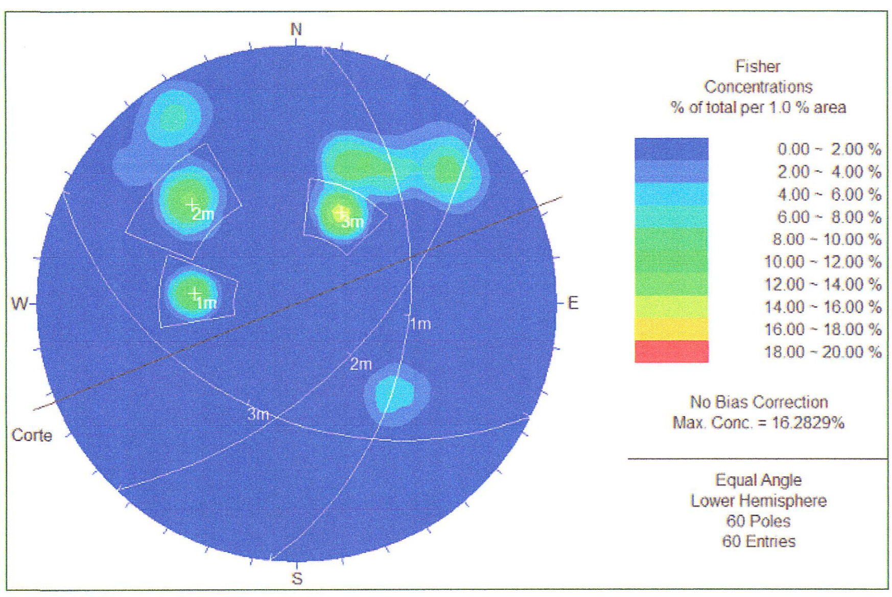
ESTACION GEOMECANICA N° 30 KM 35+548
