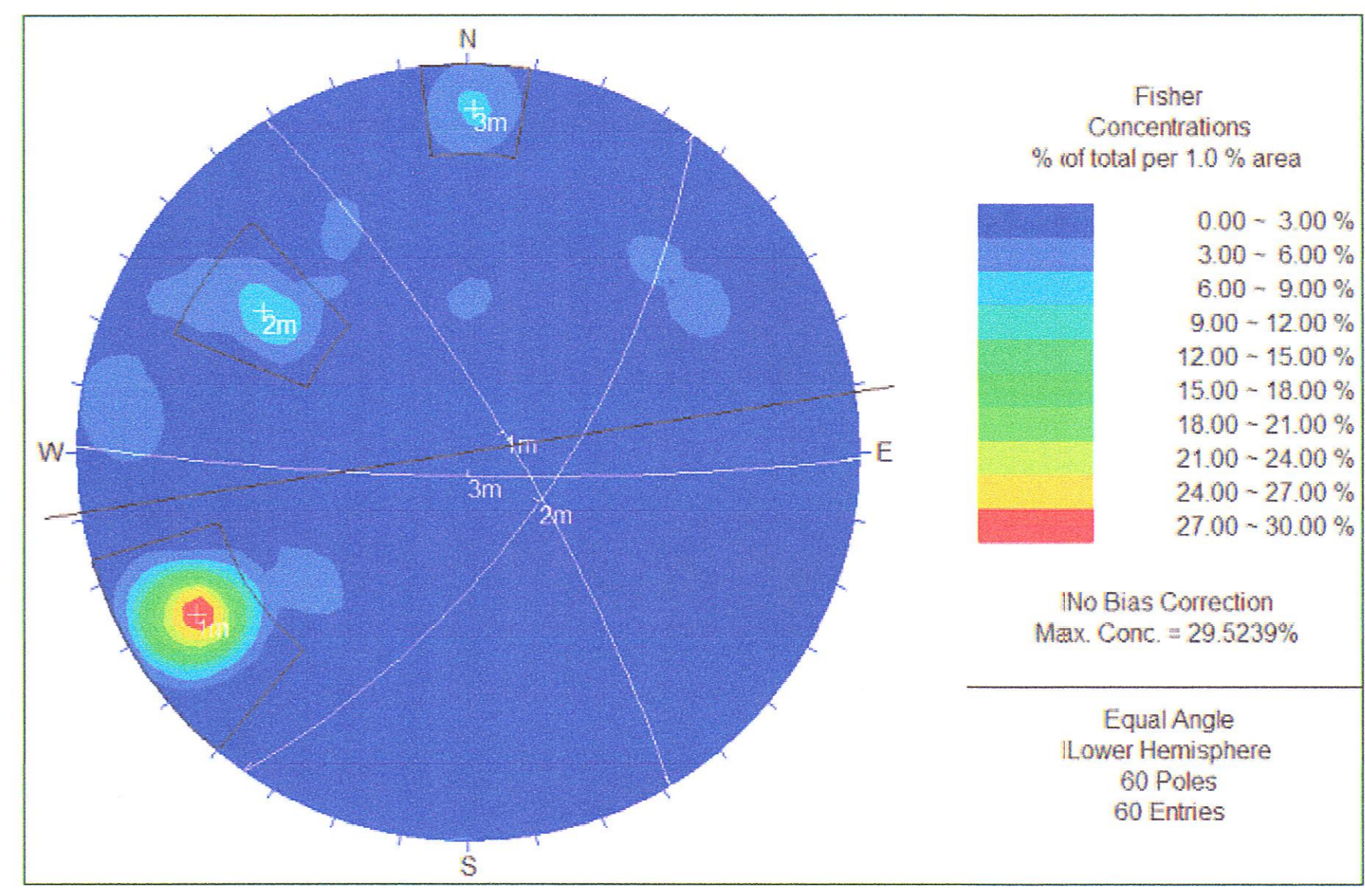
ESTACION GEOMECANICA N° 31 KM 35+698
