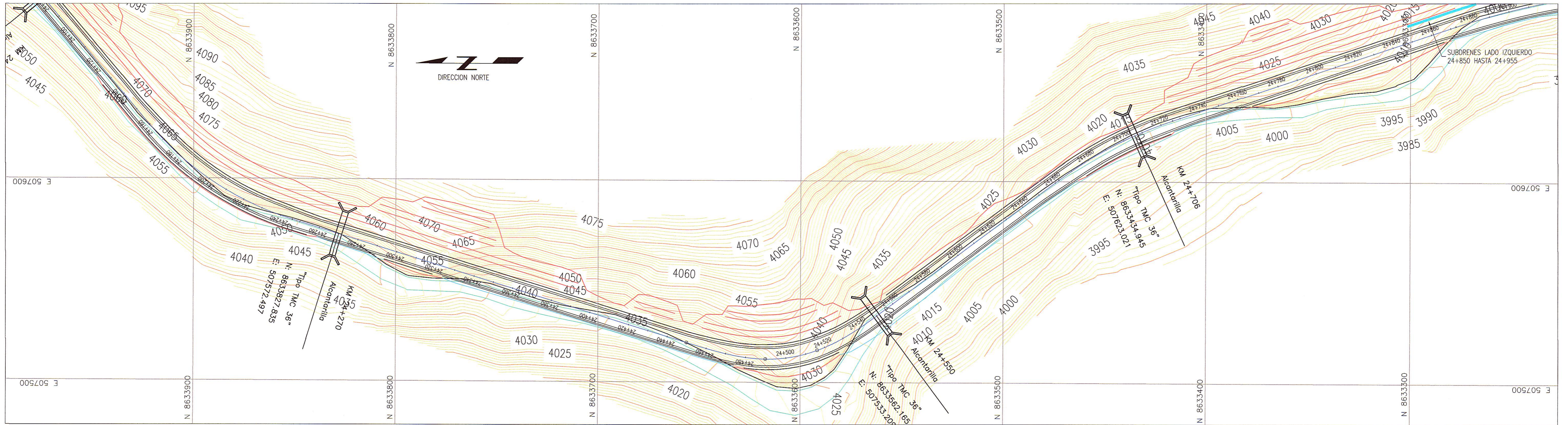
PLANTA 1:1000
