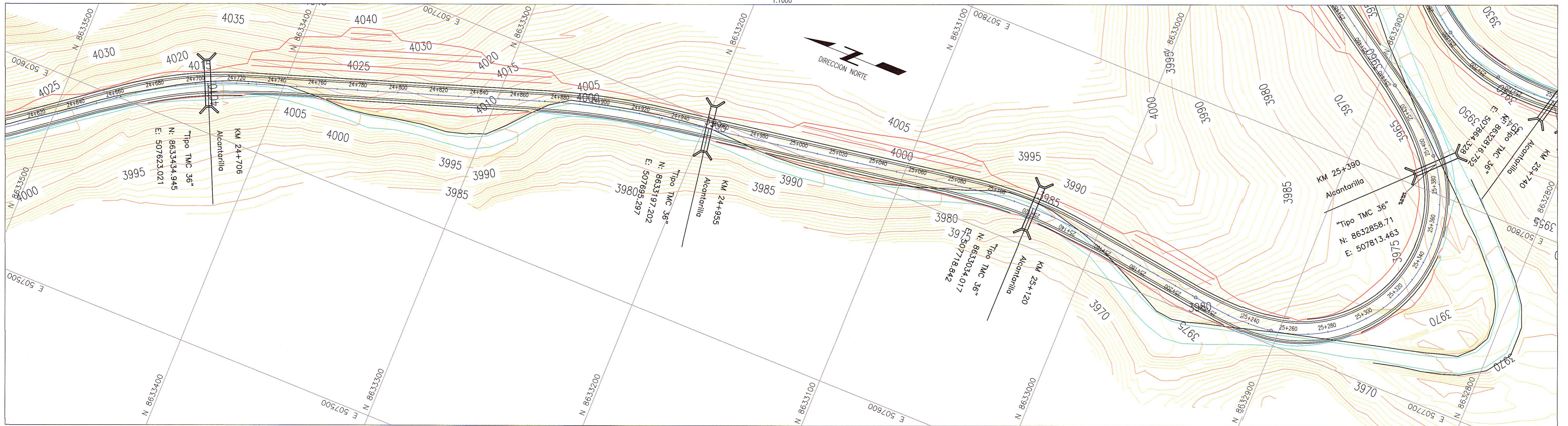
PLANTA 1:1000
