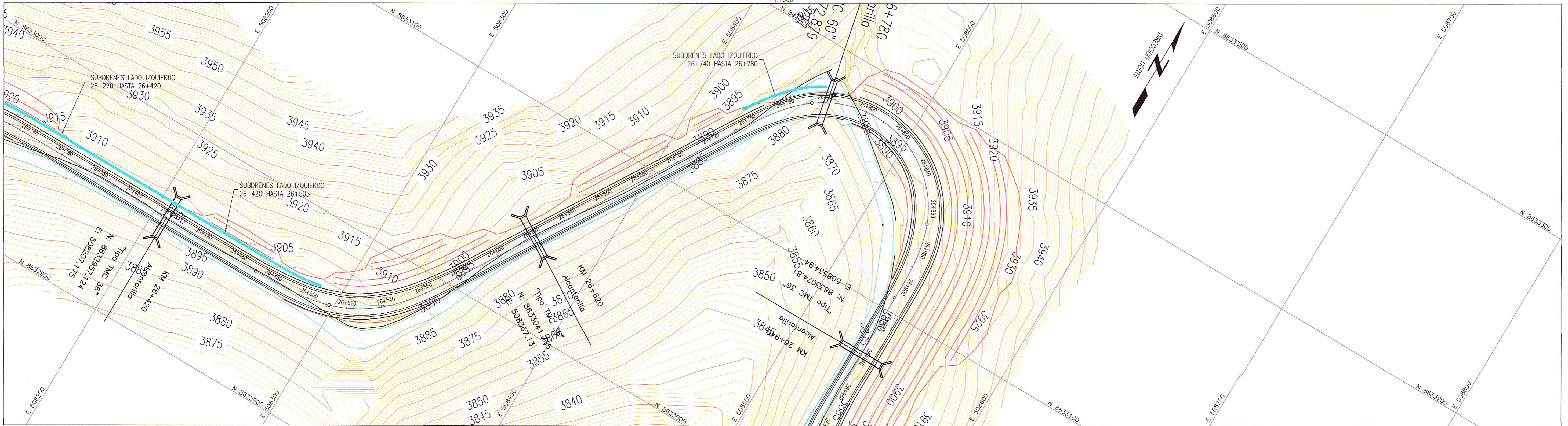
PLANTA 1:1000
