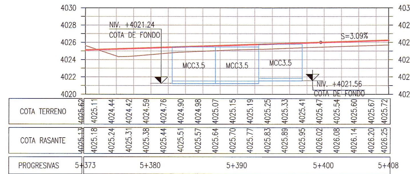
PERFIL LONGITUDINAL 1:250
