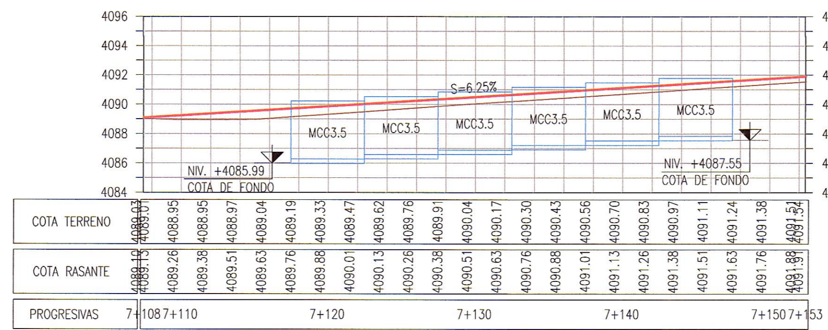
PERFIL LONGITUDINAL 1:250
