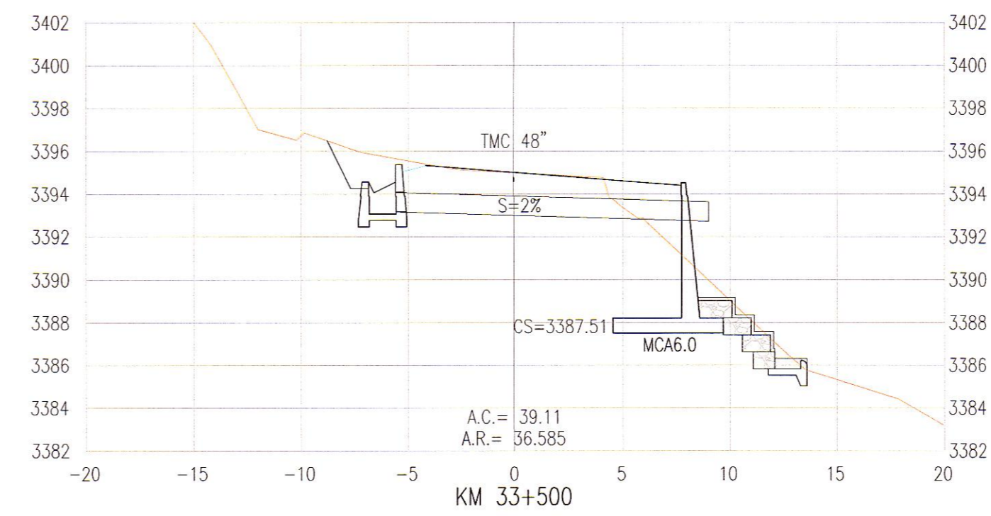
KM 33+477.5 A KM 33+507.5
