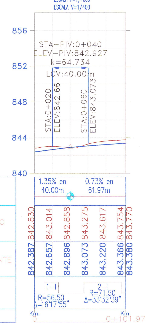
PERFIL RAMAL "C" (CALZADA-TARAPOTO) ESCALA H=1/4000 ESCALA V=1/400
