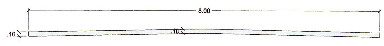
SECCIÓN TRANSVERSAL CARPETA ASFALTICA EXISTENTE ESC: 1/50
