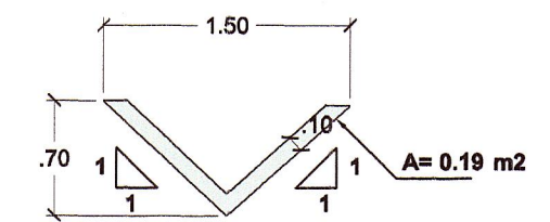
SECCIÓN TRANSVERSAL CUNETA EXISTENTE ESC: 1/50
