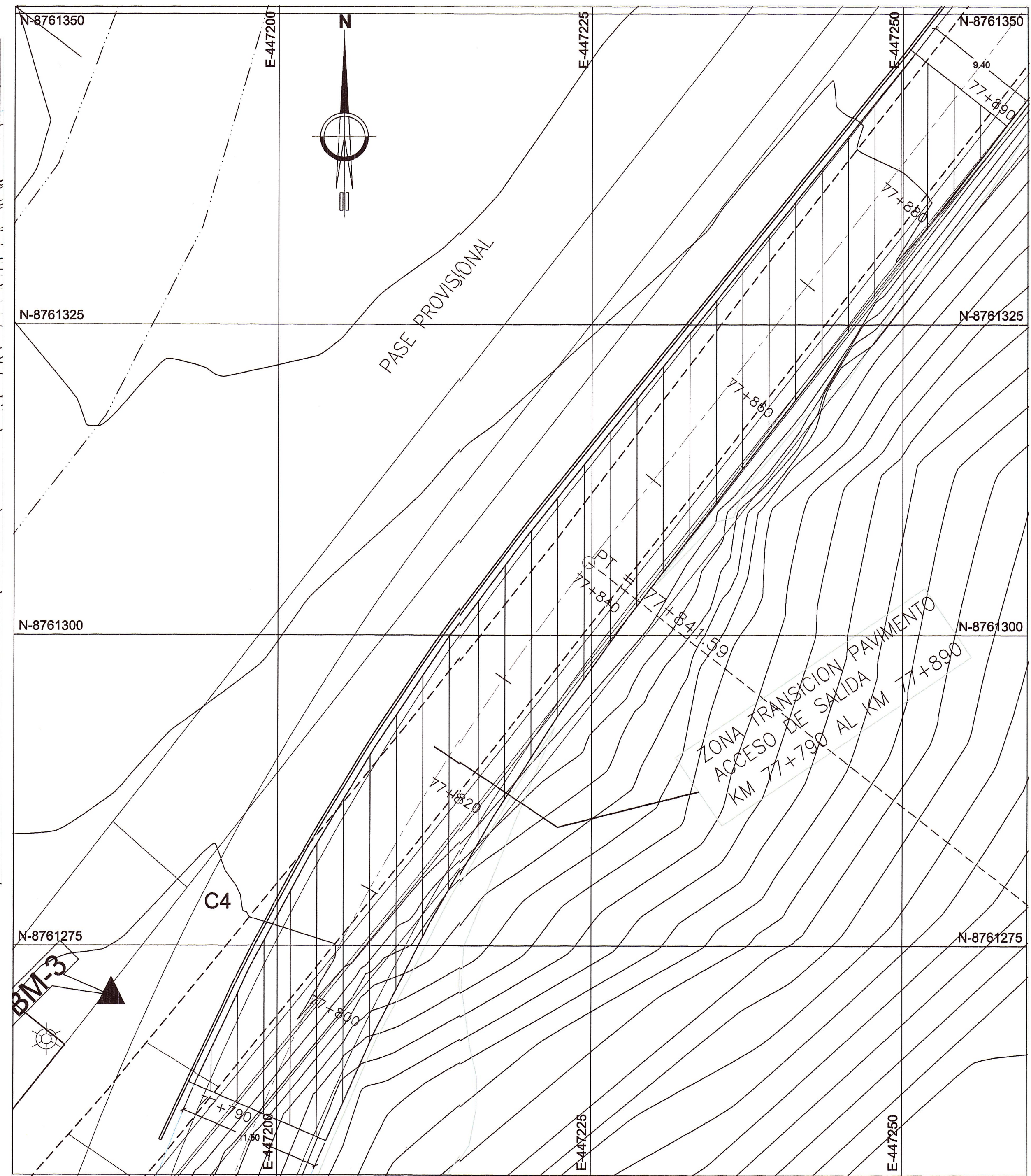
PLANTA TUNEL YANANGO ACCESO DE SALIDA ESC. 1/250
