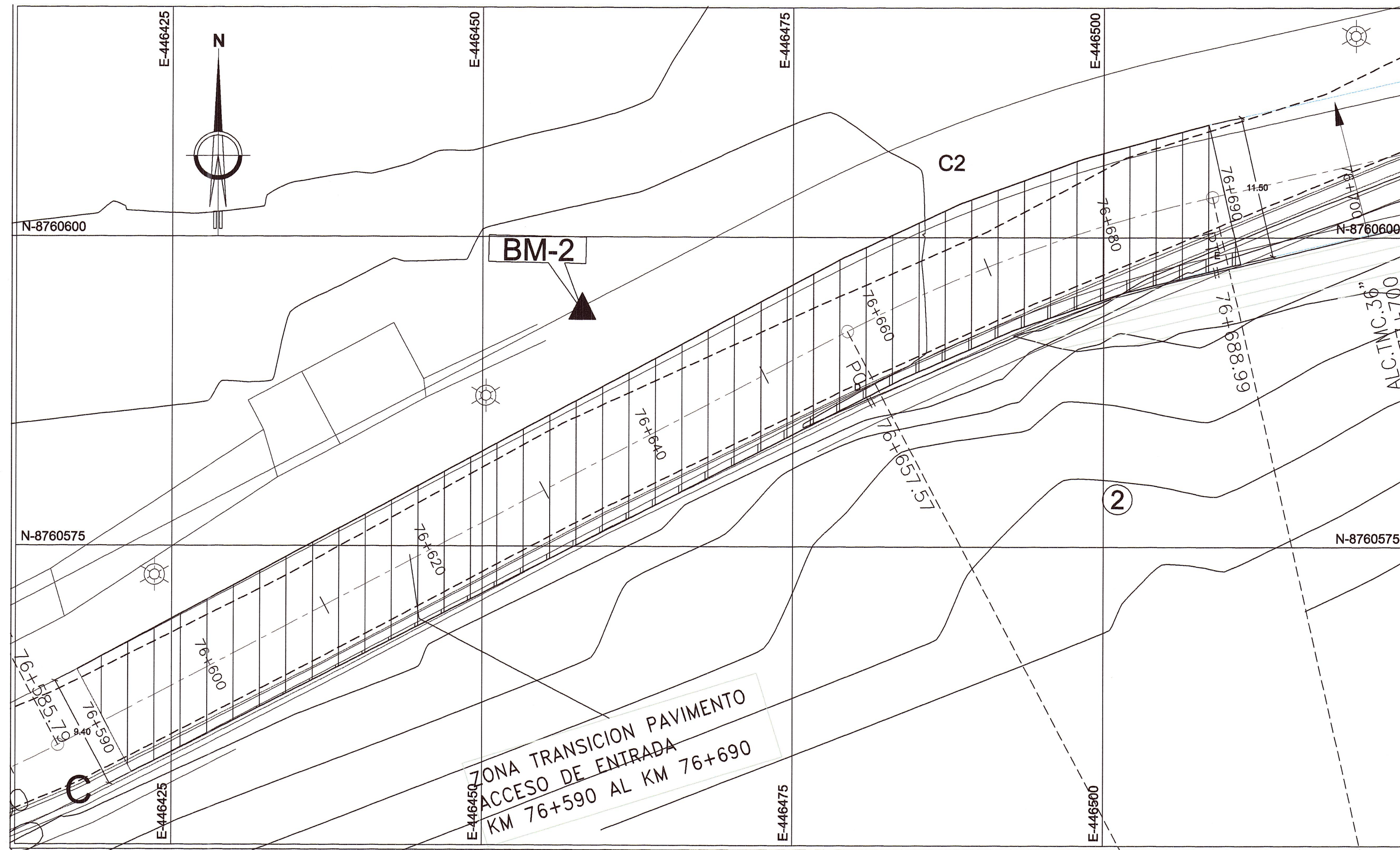
PLANTA TUNEL YANANGO ACCESO DE ENTRADA ESC. 1/250
