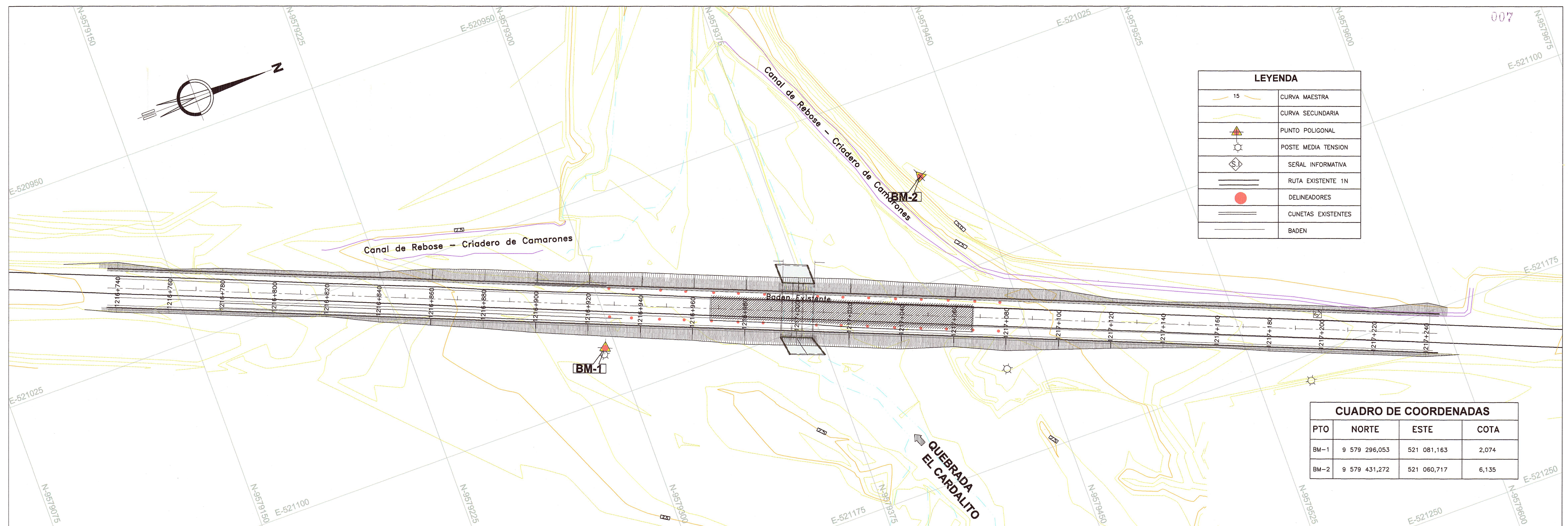
PLANTA PONTON km 1217+000 ESC. 1/750
