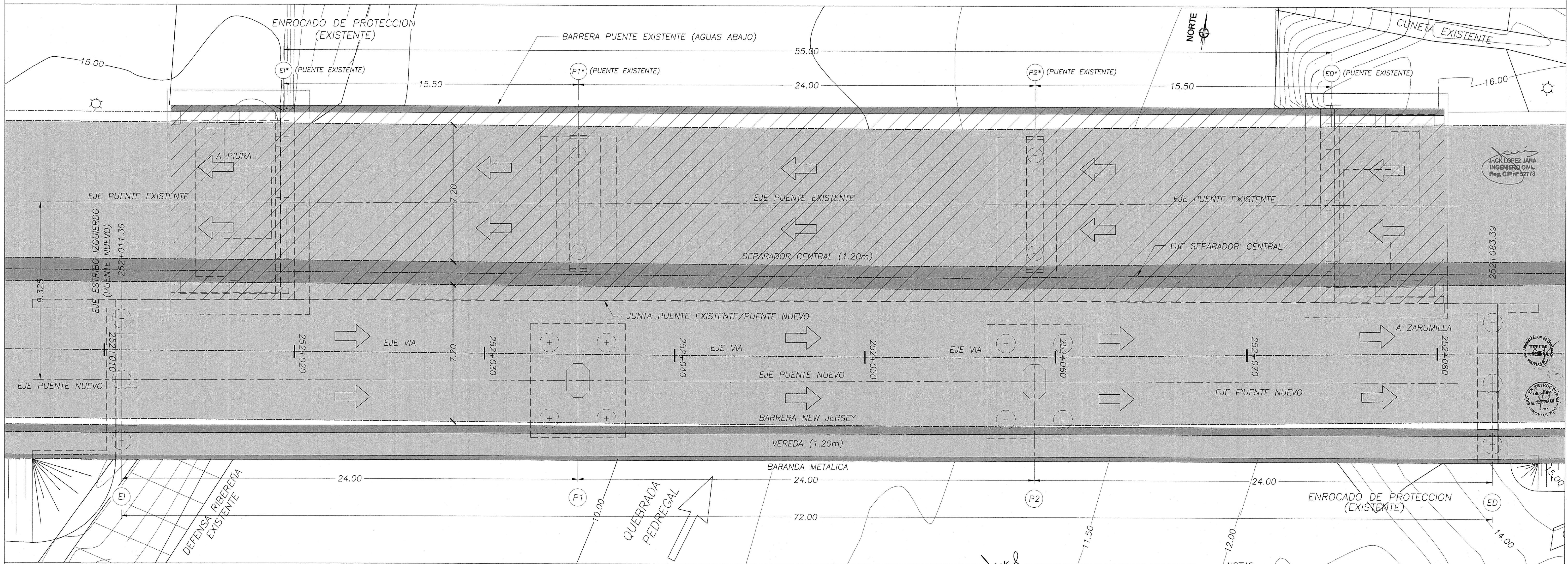
PLANTA ESC:1/200
